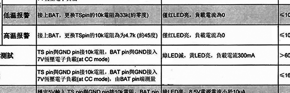
NTC 模組
