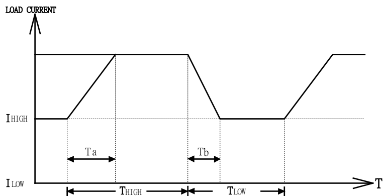
圖 5-4 動態負載電流
