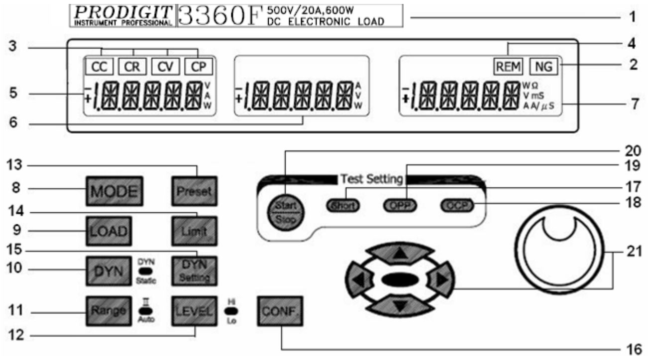
圖 3-1 3360F 系列高功率電子負載之面板圖
