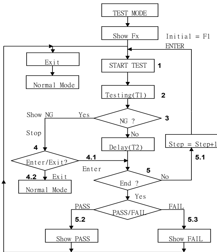
圖 3-6 測試模式操作流程圖
