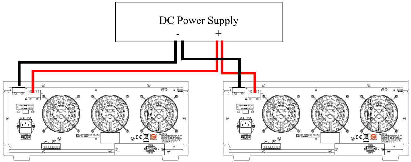
圖 5-10 電子負載多組並聯之連接圖
