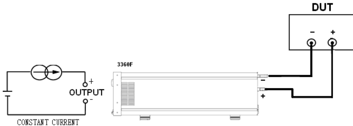
圖 5-8 固定電流源之連接圖
