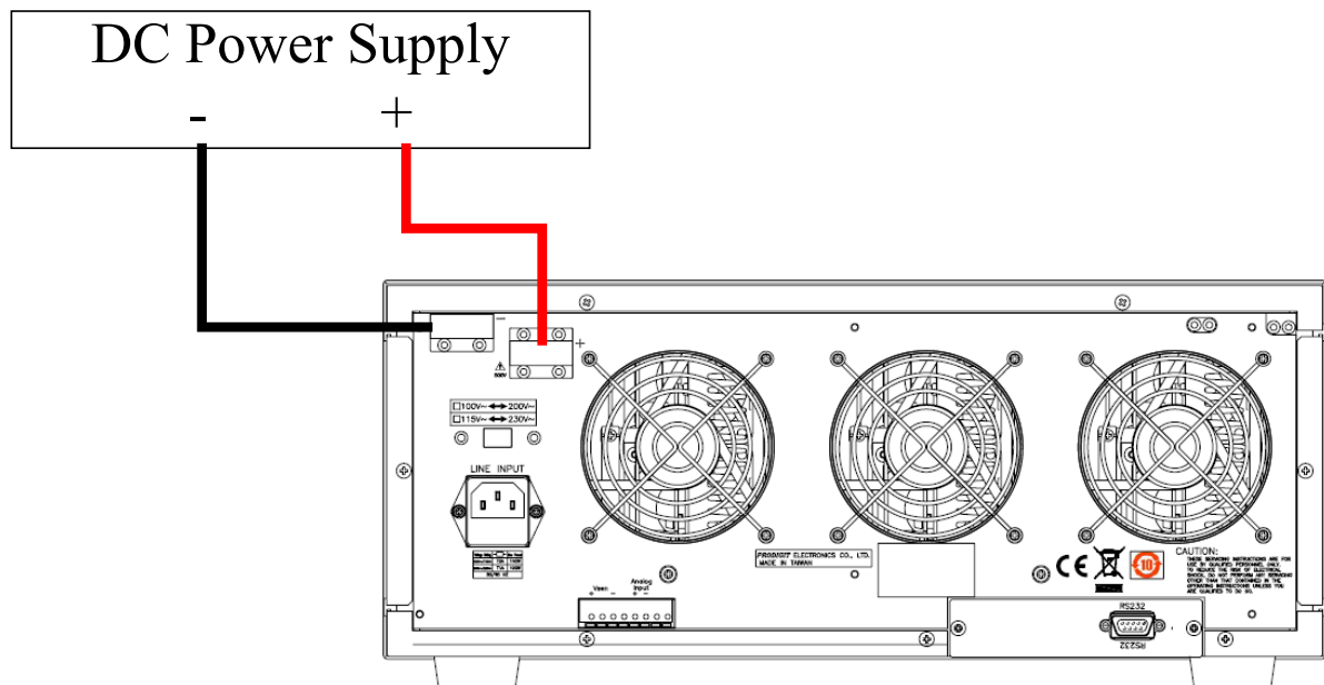
圖 5-1 本地電壓檢知連接圖
