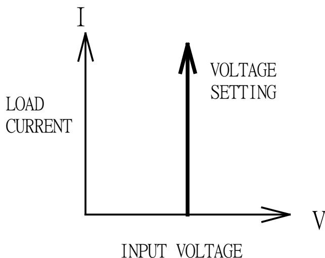
圖 1-7 固定電壓模式特性圖
