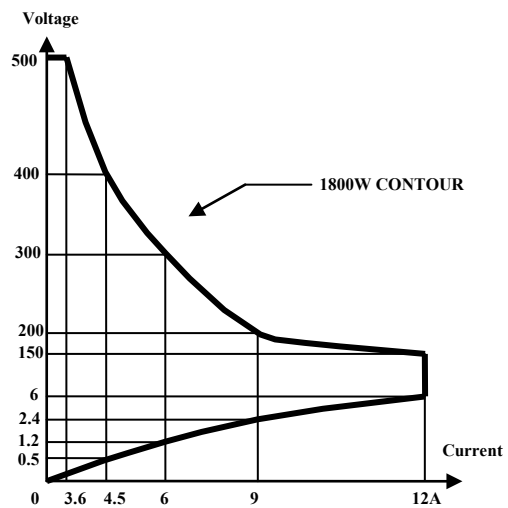
圖 1-4 3367F 高功率電子負載功率曲線圖
