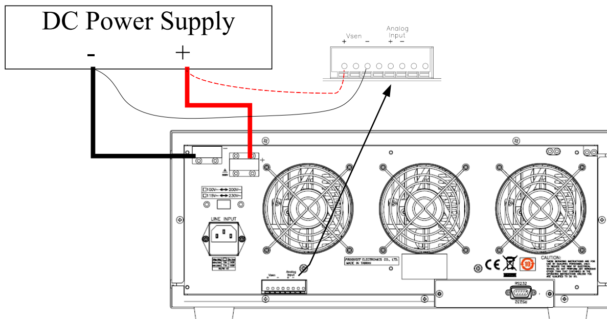
圖 3-3 典型 3360F 系列高功率電子負載連接方式
