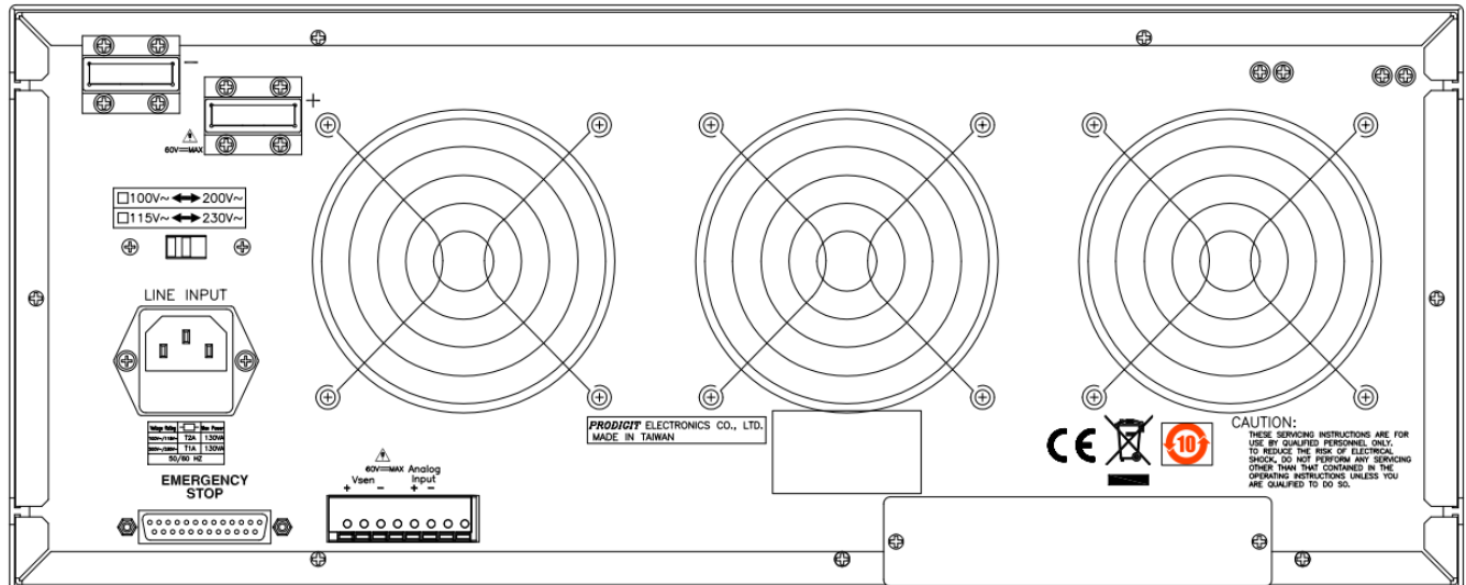
圖 2-10 3360F 系列背面
