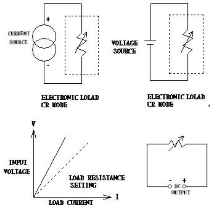
圖 5-6 固定電阻操作模式之應用
