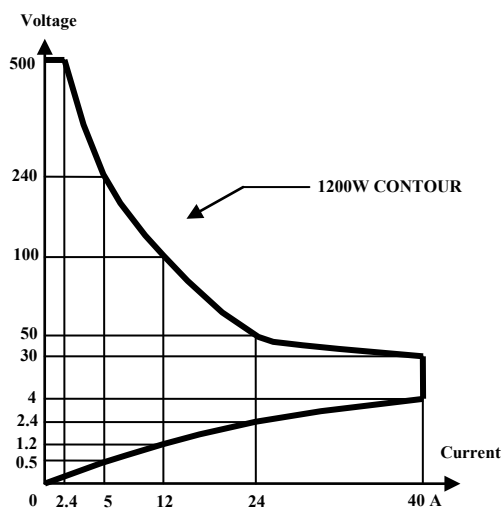
圖 1-2 3361F 高功率電子負載功率曲線圖
