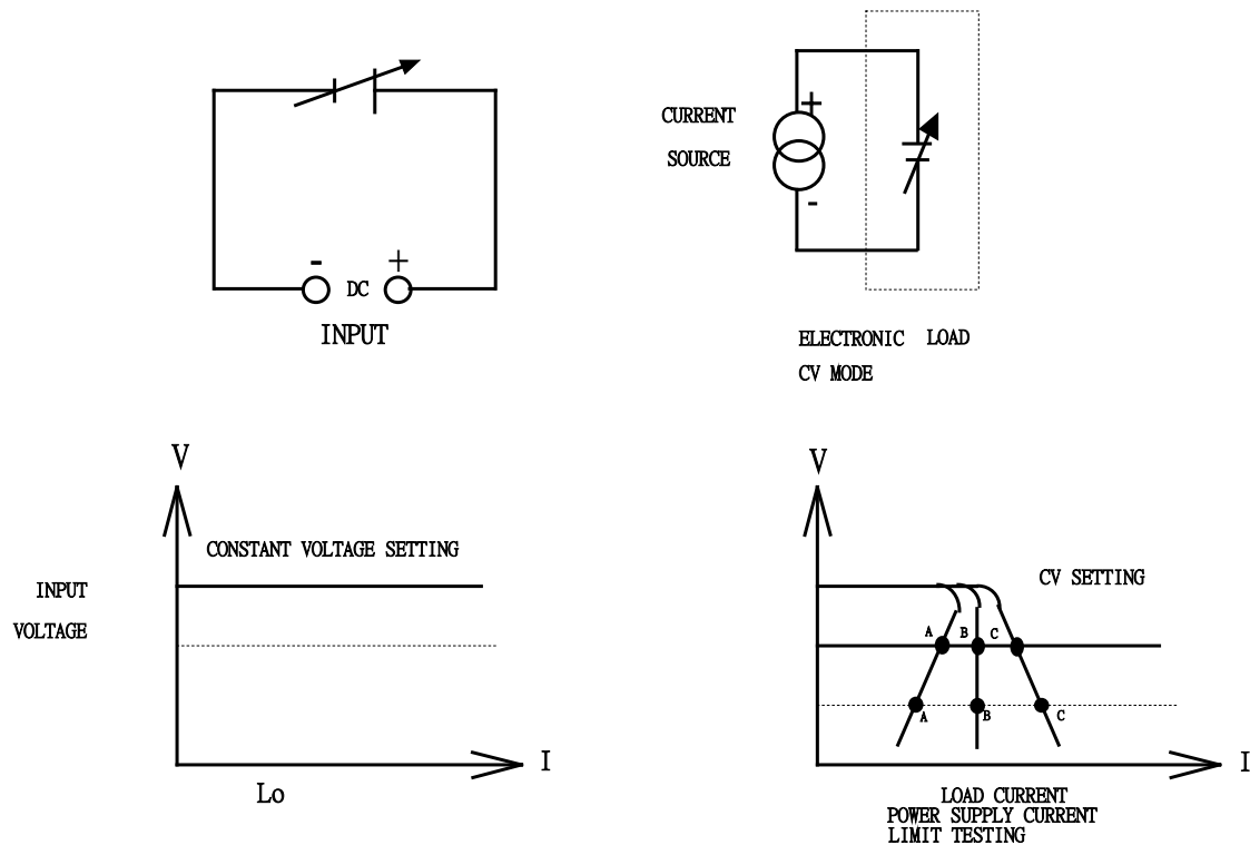
圖 5-5 固定電壓操作模式之應用
