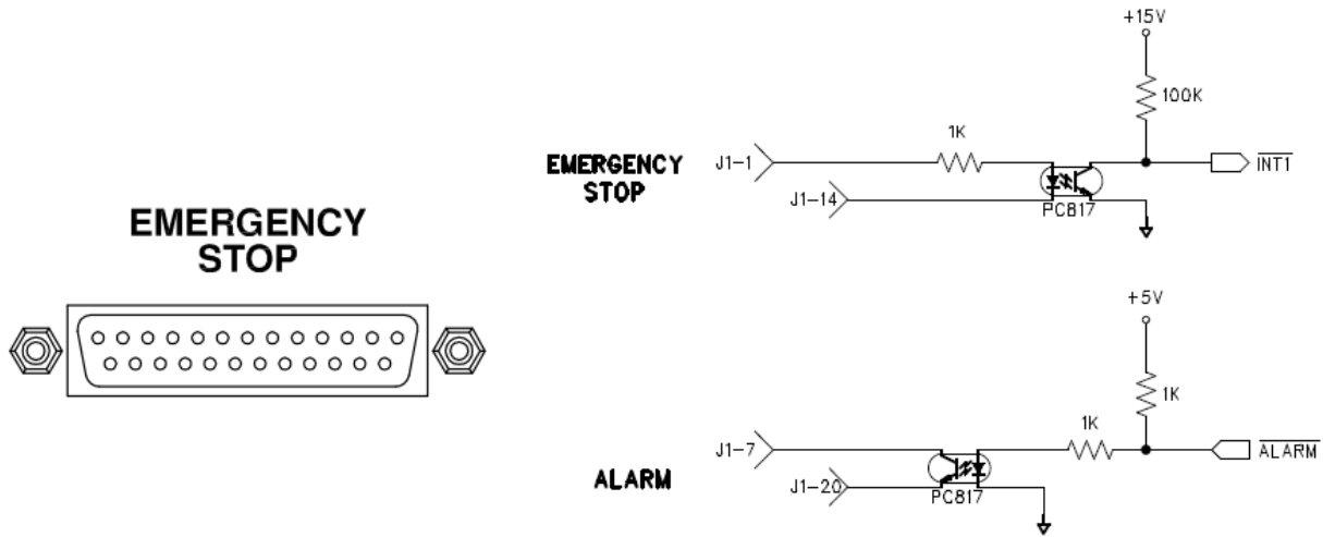
圖 2-9 緊急開關聯接器
