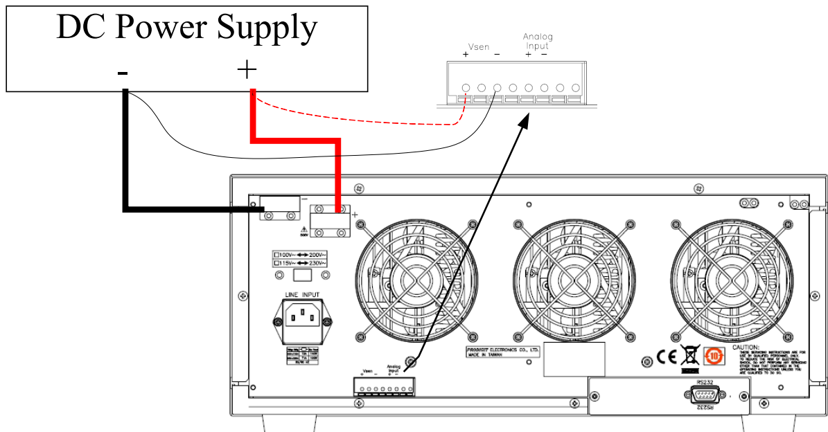
圖 5-2 遠地電壓檢知連接圖
