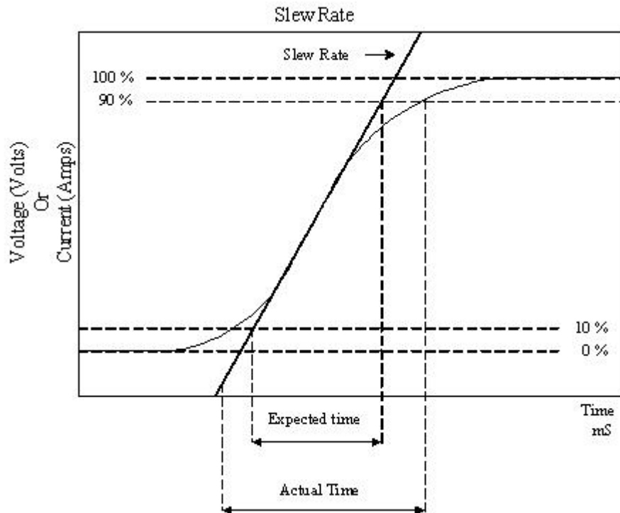
回轉率(Slew Rate)曲線圖
