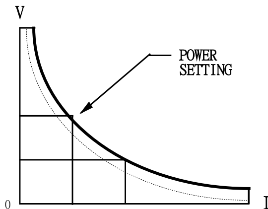
圖 1-8 固定功率模式特性圖
