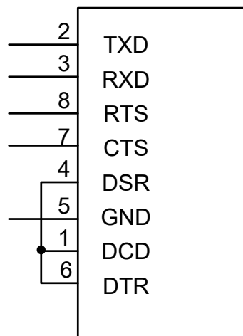
圖 4-1 後面板 RS-232C 介面連接圖
