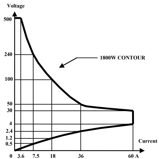
圖 1-3 3362F 高功率電子負載功率曲線圖
