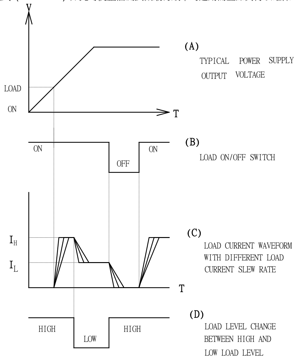
圖 2-8 負載電流波形與 LOAD ON/OFF 開關，負載準位與電源供應器之輸出電壓間的關係圖
