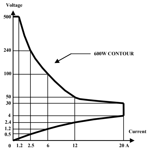
圖 1-1 3360F 高功率電子負載功率曲線圖
