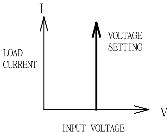
圖 1-9 固定電壓模式特性圖
