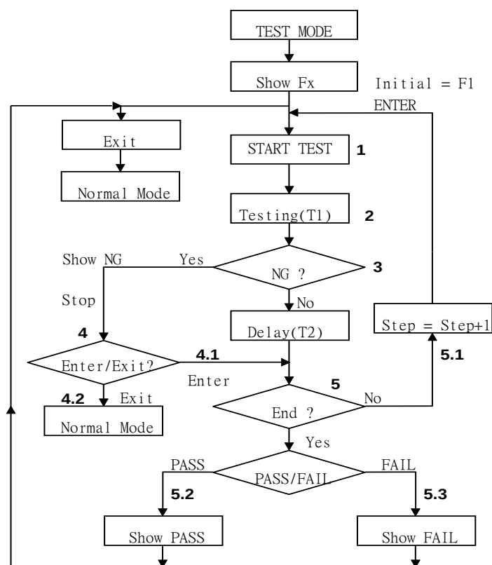
圖 3-10 測試模式操作流程圖
