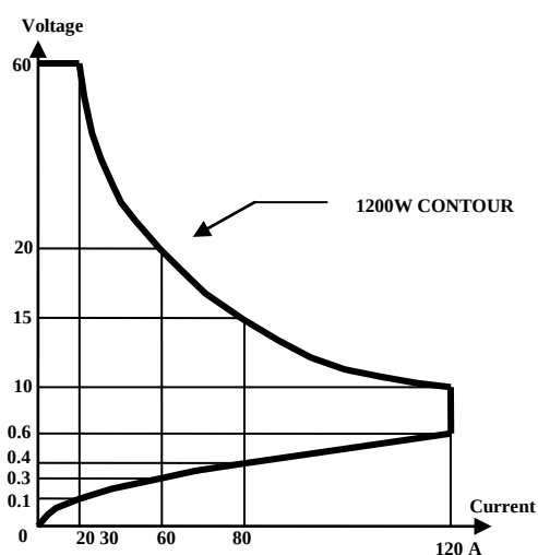
圖 1-1 3350F 高功率電子負載功率曲線圖
