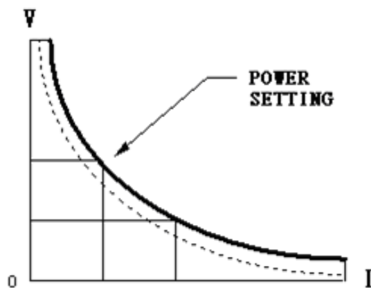
圖 1-10 固定功率模式特性圖
