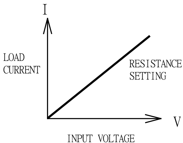
圖 1-8 固定電阻模式特性圖
