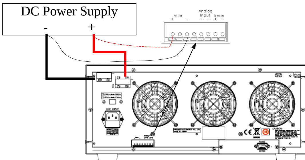
圖 3-3 典型 3350F高功率電子負載連接方式
