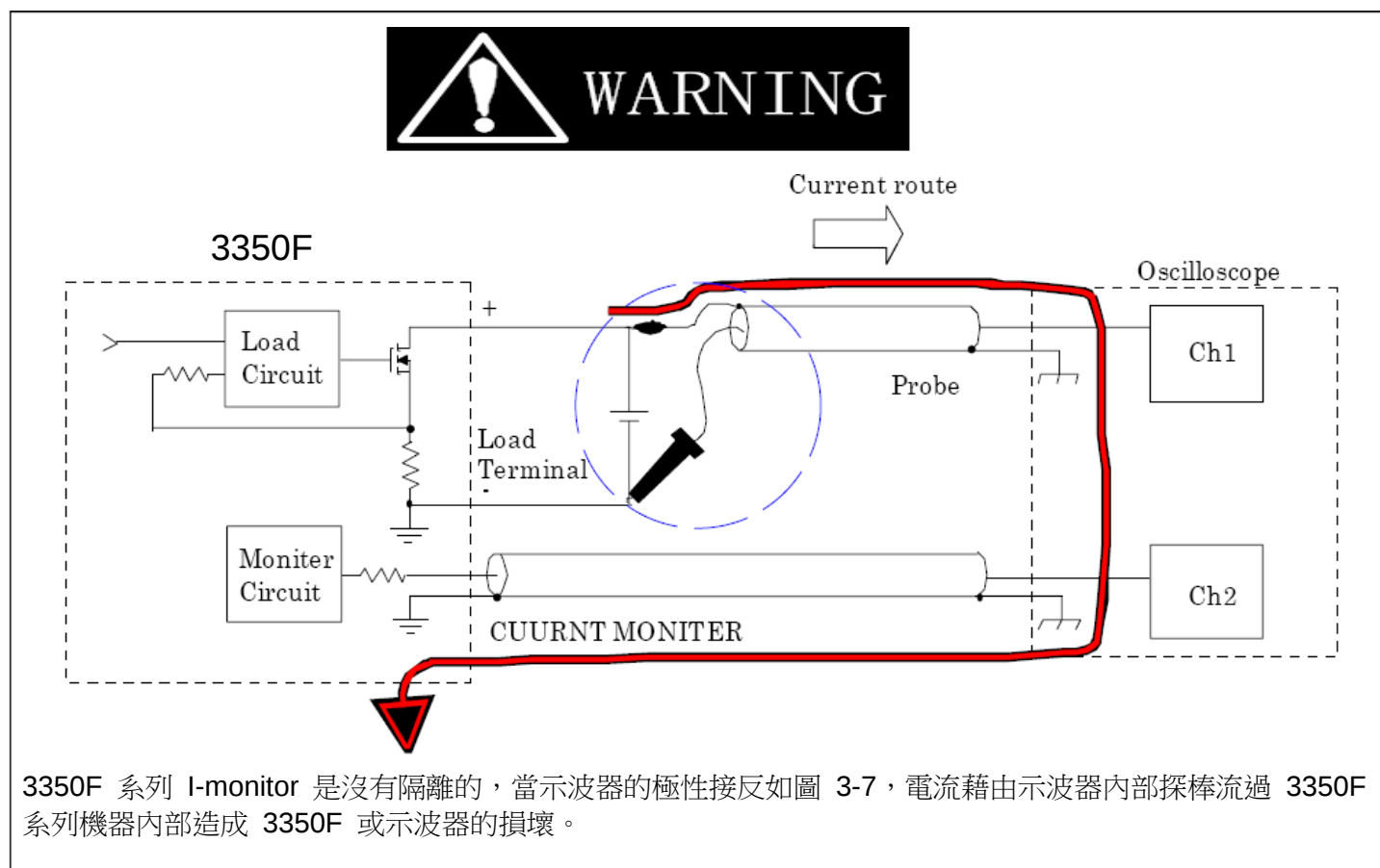
圖 3-7 示波器錯誤的連接圖
