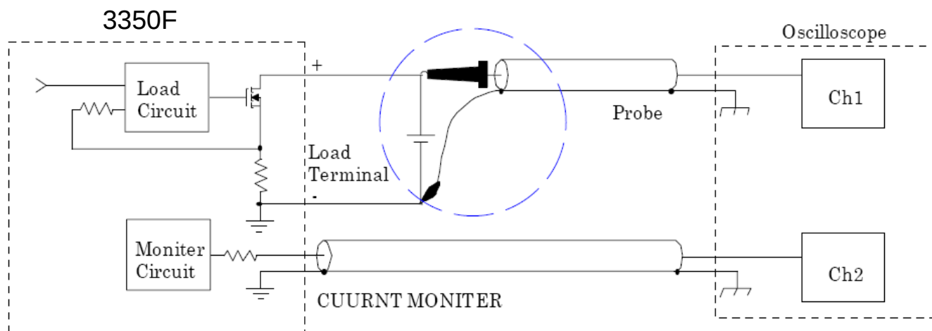
圖 3-6 示波器正確的連接圖
