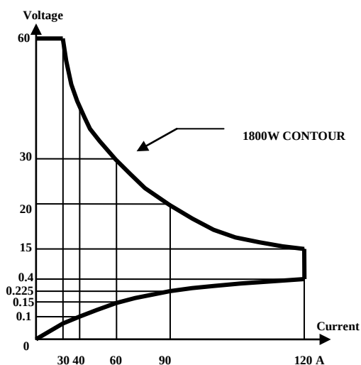
圖 1-2 3351F 高功率電子負載功率曲線圖
