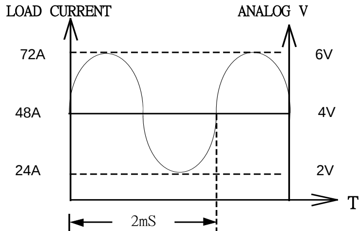
圖 3-8 負載電流之類比設定輸入
