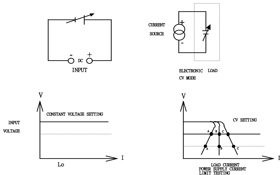
圖 5-5 固定電壓操作模式之應用
