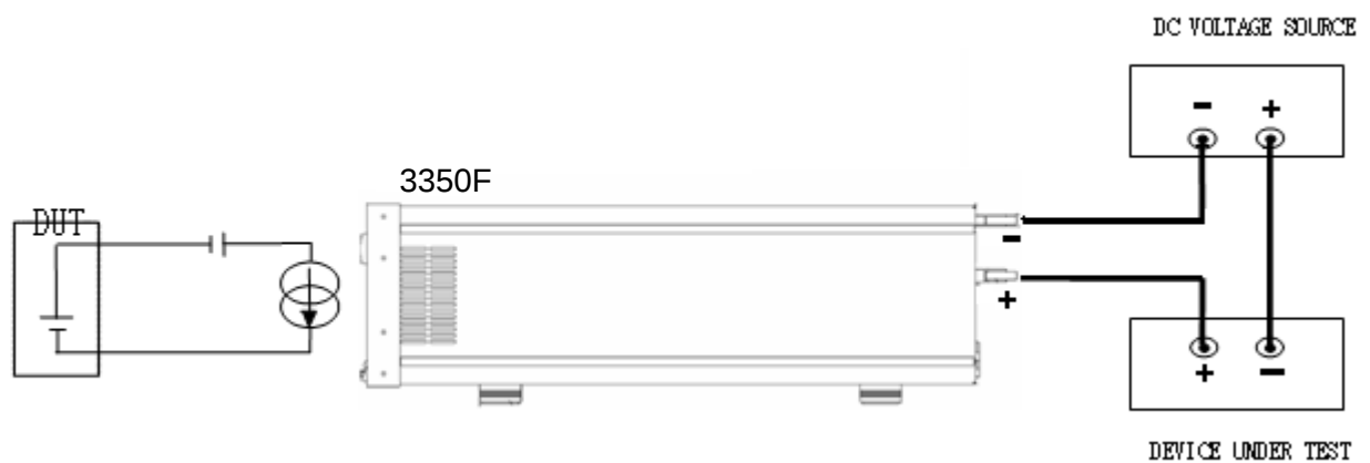
圖 5-9 高功率電子負載最低工作電壓為 0V 時的連接圖
