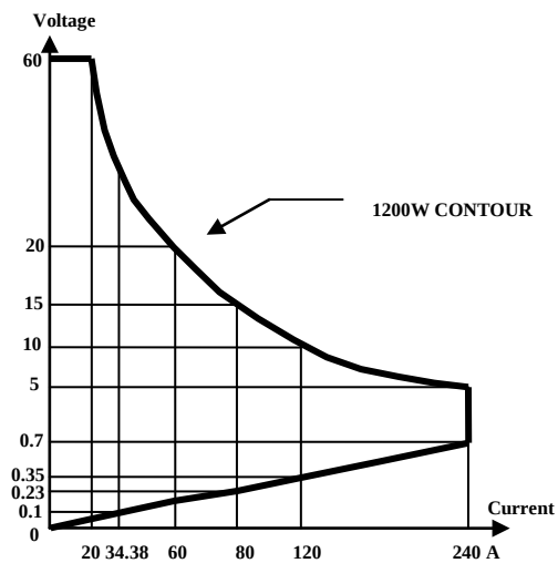
圖 1-3 3352F 高功率電子負載功率曲線圖
