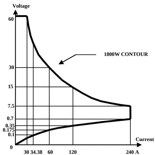
圖 1-4 3353F 高功率電子負載功率曲線圖
