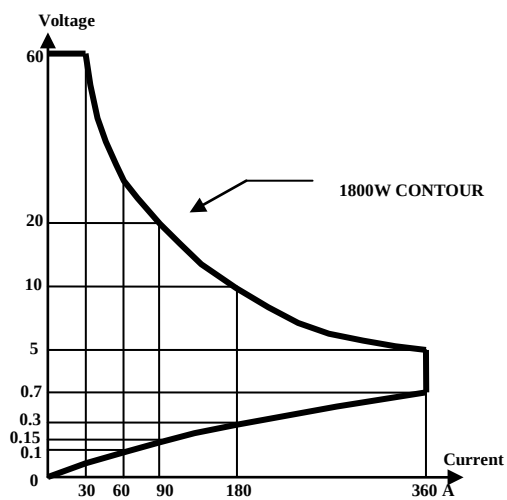
圖 1-5 3354F 高功率電子負載功率曲線圖
