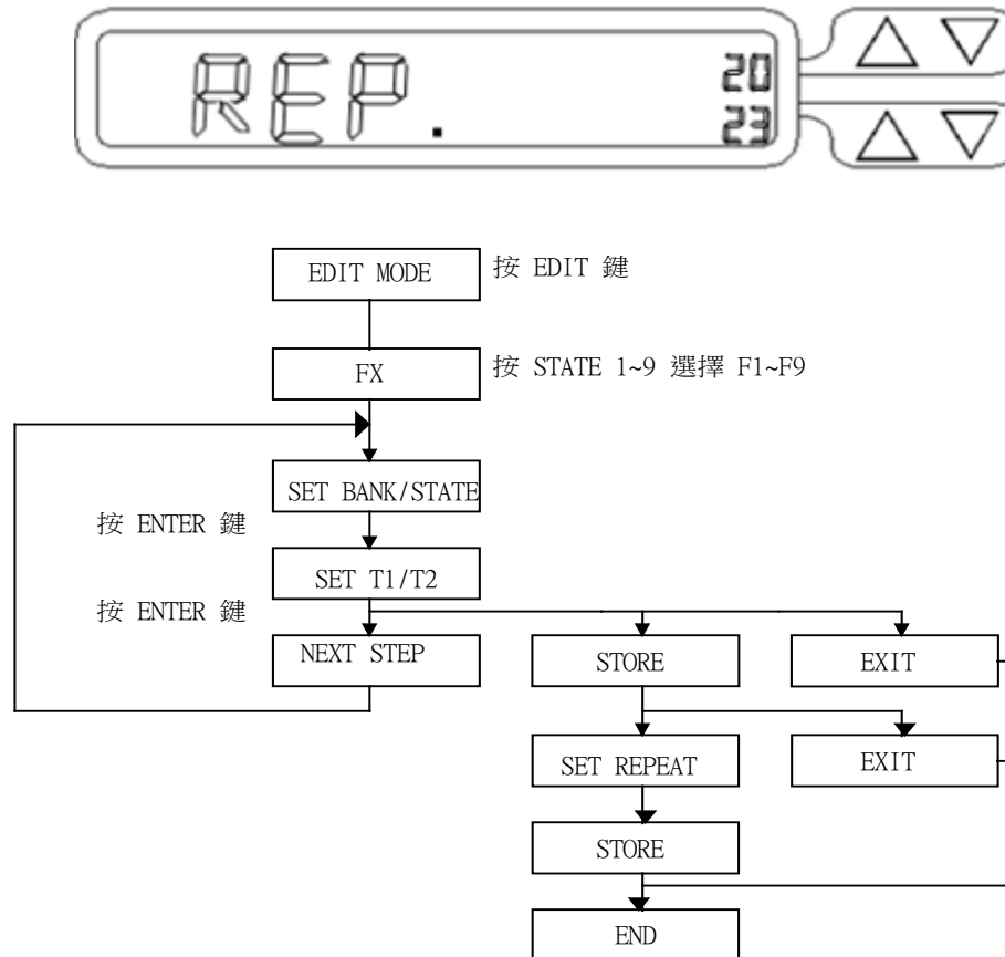
圖 3-9 編輯模式操作流程圖
