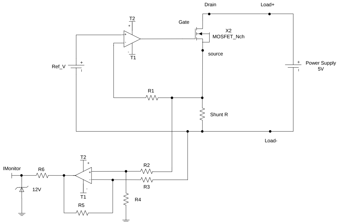
圖 3-5 3350F 系列 I-monitor 等效電路圖
