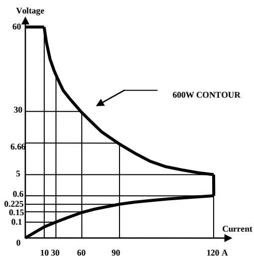
圖 1-6 3356F 高功率電子負載功率曲線圖
