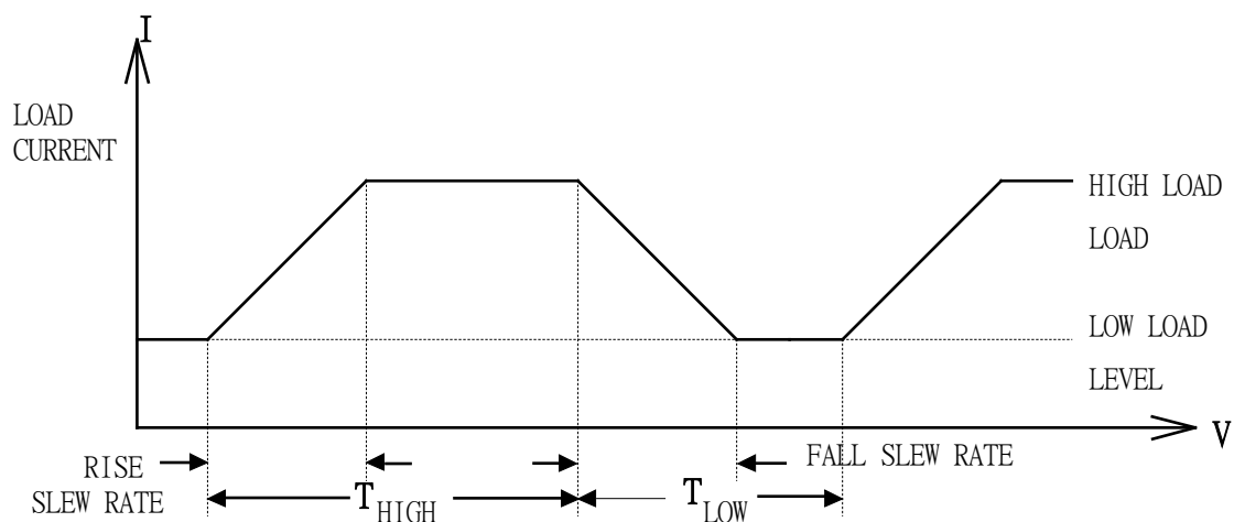
圖 1-11 動態負載電流波形圖
