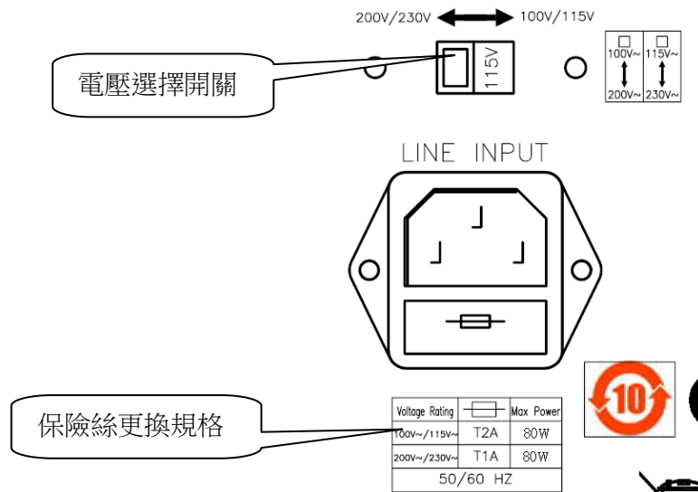
圖 2-1 電源設定圖
