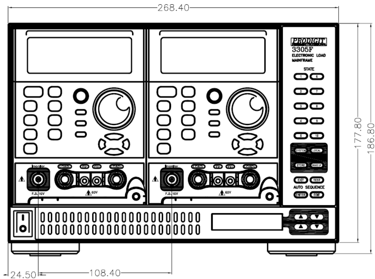
圖 3-1 3305F 前面板圖
