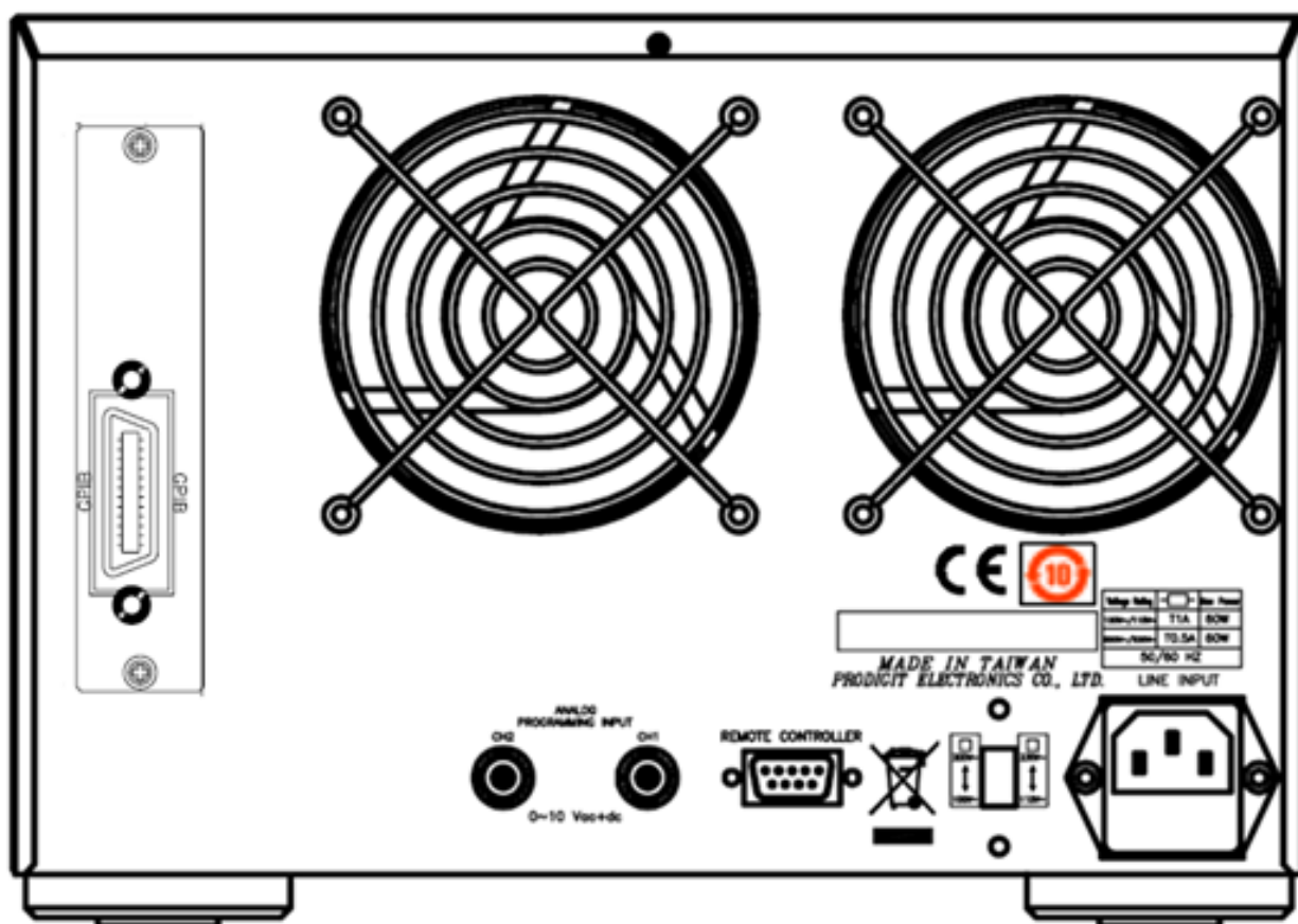
圖 3-3 3305F 後面版圖
