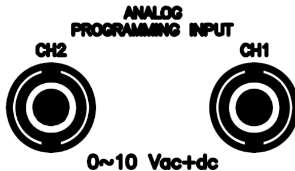
圖 2-10 3305F 類比信號設定輸入介面
