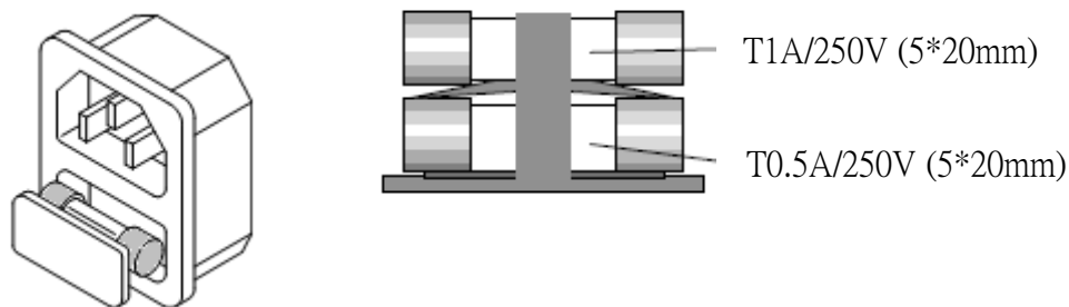
圖 2-2 保險絲座
