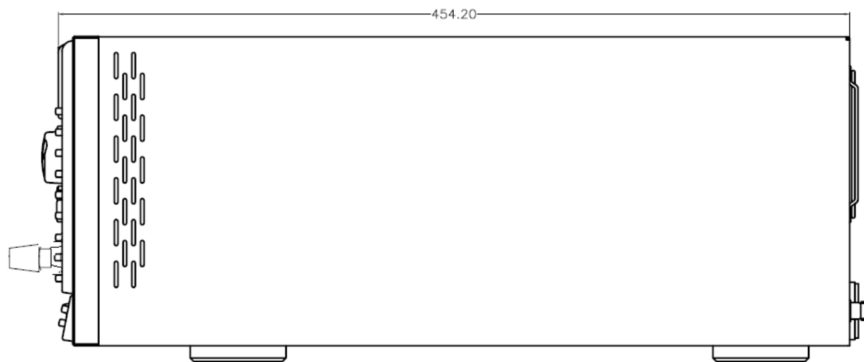
圖 3-2 3302F 側面圖
