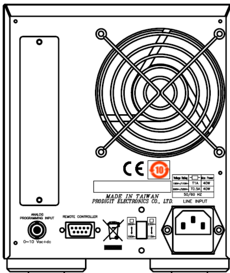
圖 3-3 3302F 後面板圖
