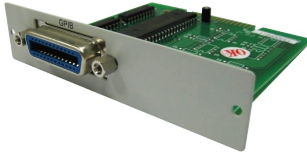
圖 2-5 3300F GPIB 連接埠圖
