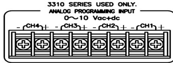
圖 2-10 3300F 類比信號設定輸入介面
