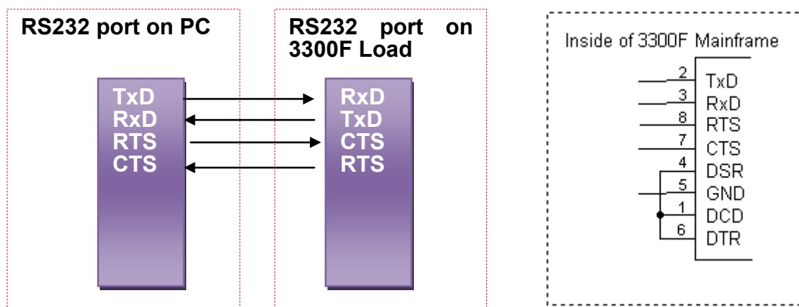
圖 4-1 後面板 RS232 介面連接圖
