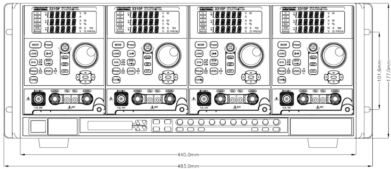
圖 3-1 3300F 前面板圖
