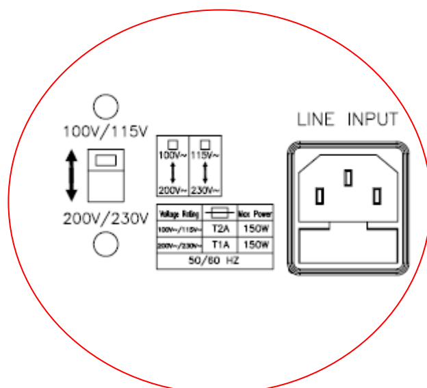
圖 2-1 電源設定圖
