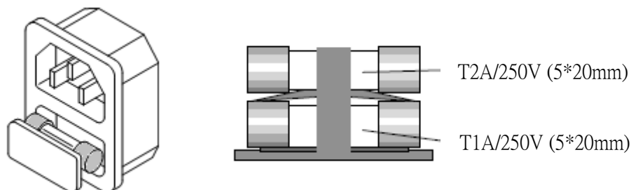
圖 2-2 保險絲座
