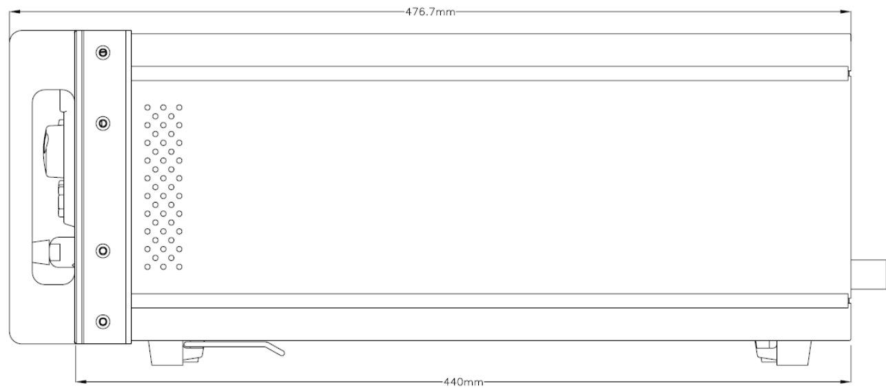
圖 3-2 3300F 側面圖
