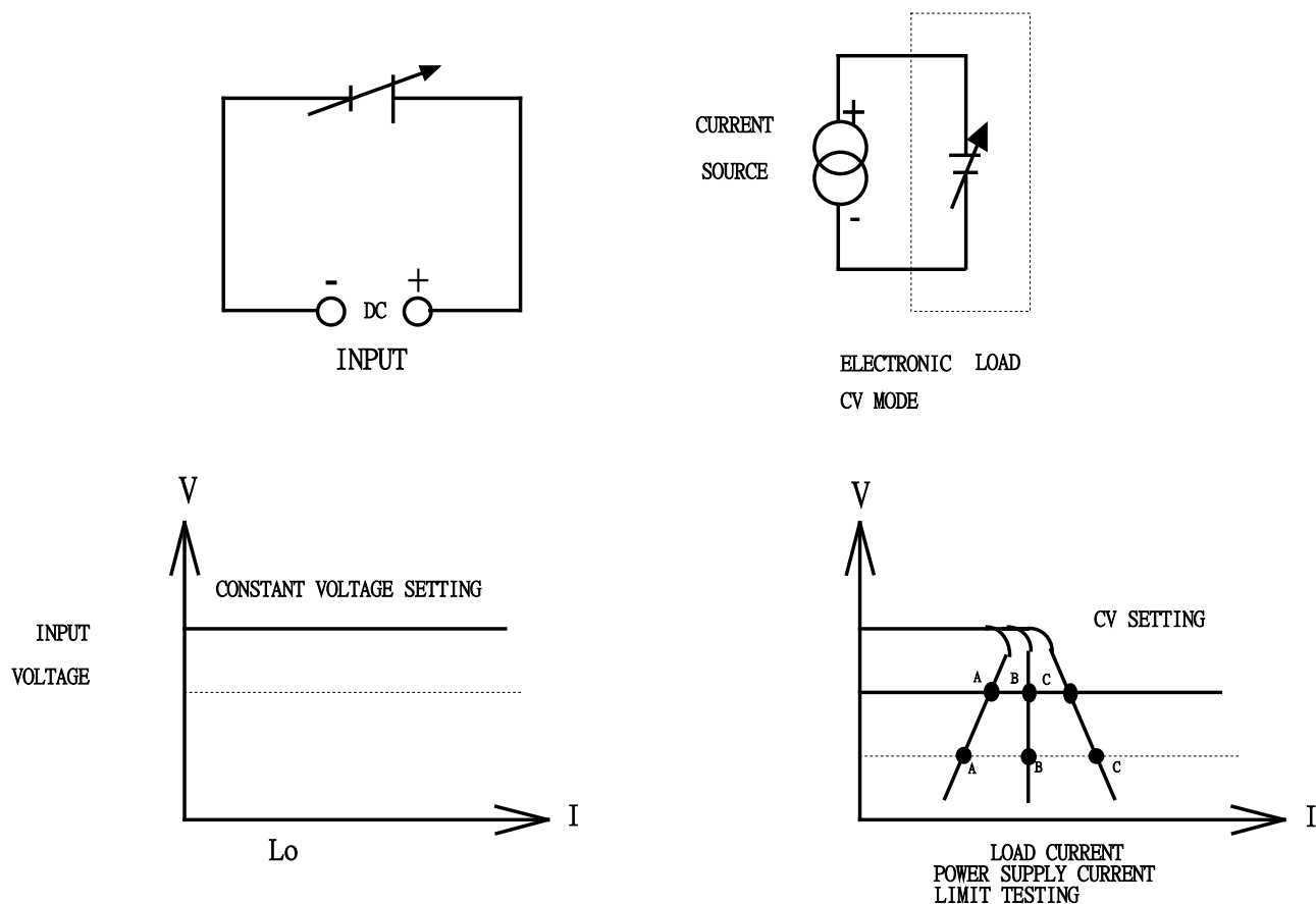
圖 4-6 固定電壓操作模式之應用
