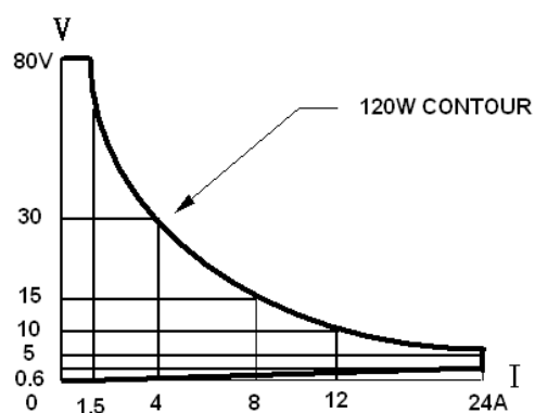
圖 1-3 3332F 0-80V/0-24A 120W 電子負載功率曲線圖
