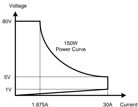
圖 1-5 3337F 0-80V/0-30A 150W 電子負載功率曲線圖
