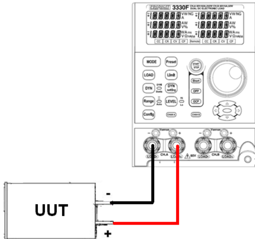
圖 4-1 本地電壓檢知連接圖
