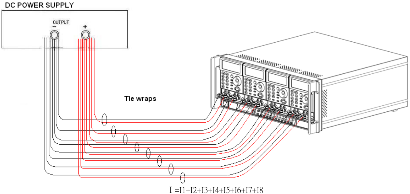
圖 4-9 電子負載多組並聯之連接圖
