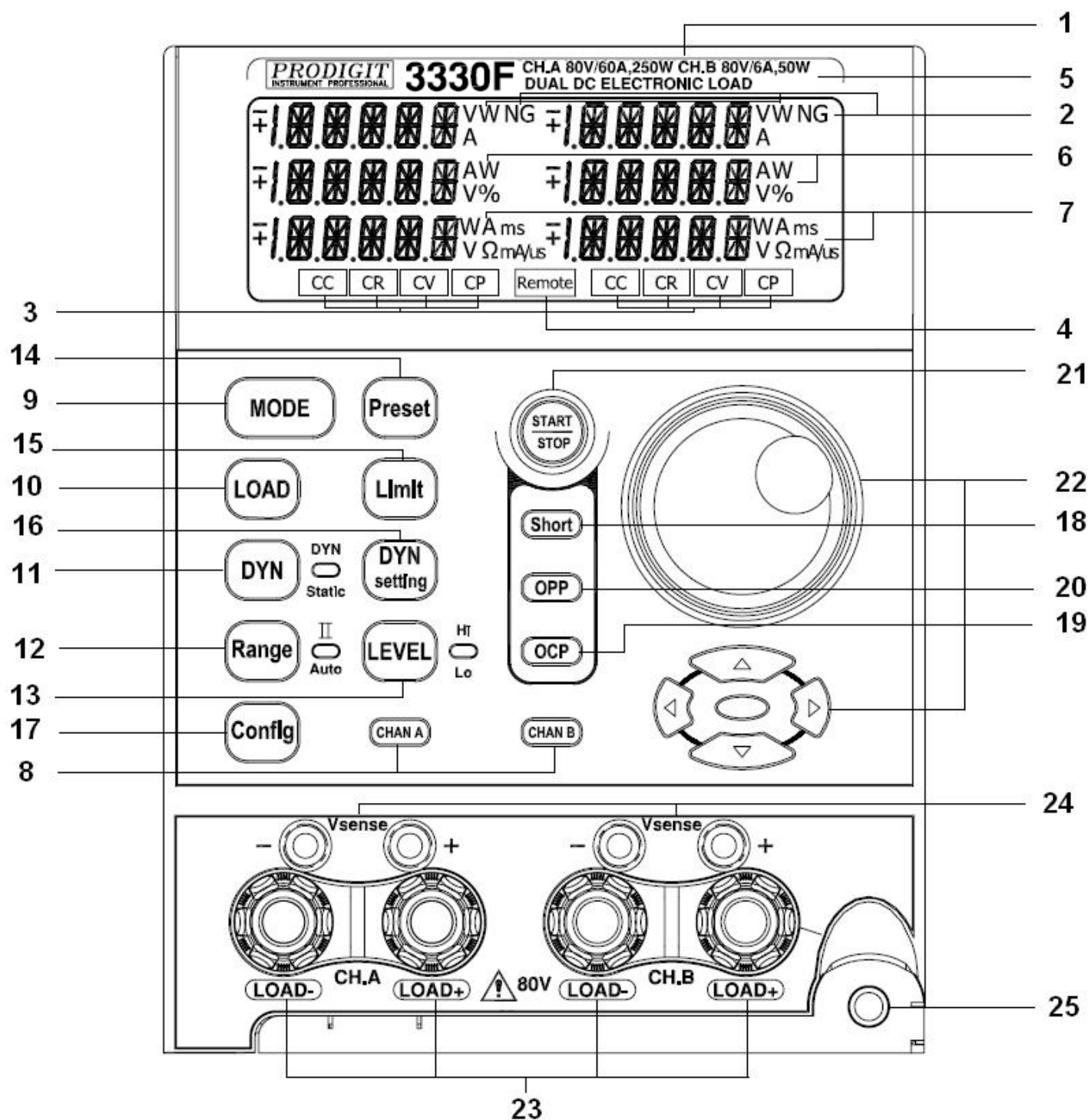
圖 3-1 前面板圖
