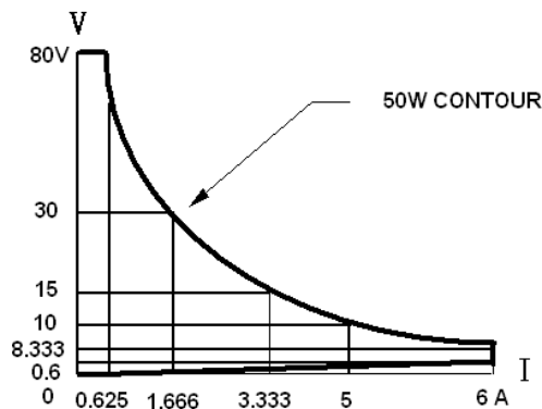
圖 1-2 3330F CHB 0-80V/0-6A 50W 電子負載功率曲線圖
