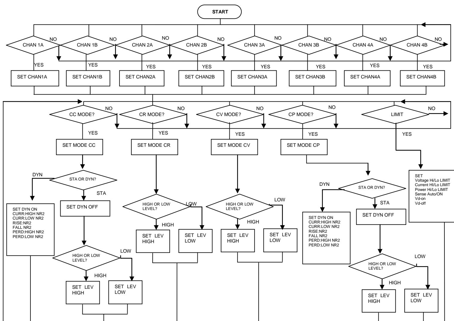
圖 2-3 3330F 系列電子負載操作流程圖
