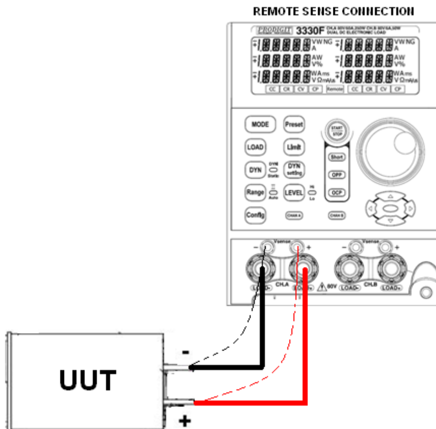
圖 4-2 遠地電壓檢知連接圖
