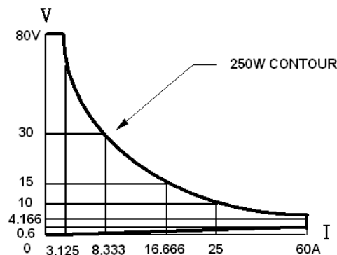
圖 1-1 3330F CHA 0-80V / 0-60A 250W 電子負載功率圖
