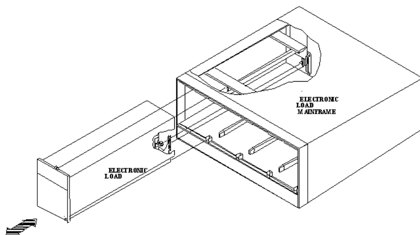
圖 2-2 電子負載裝入及拔出
