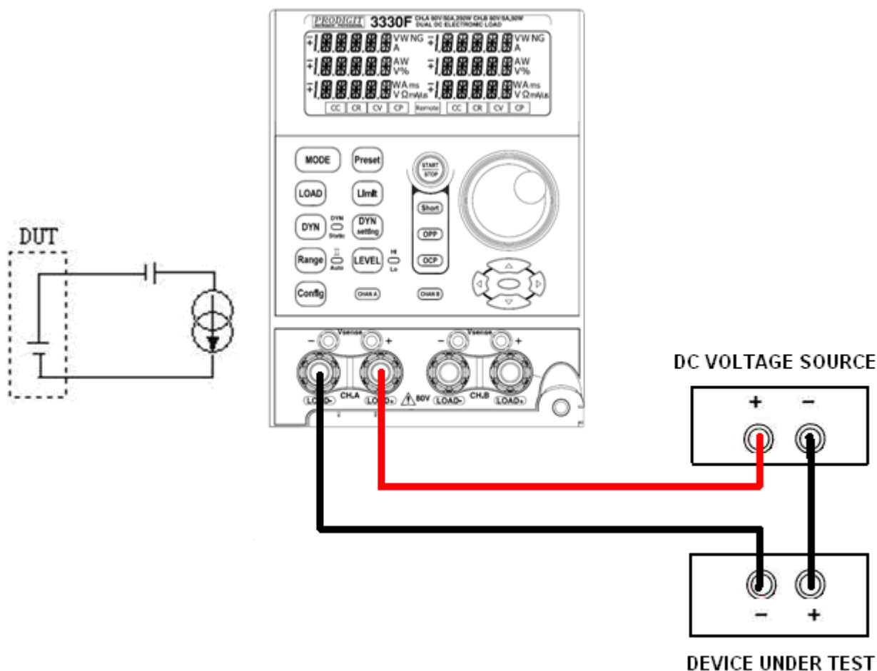
圖 4-10 高功率電子負載最低工作電壓為 0V 時的連接圖
