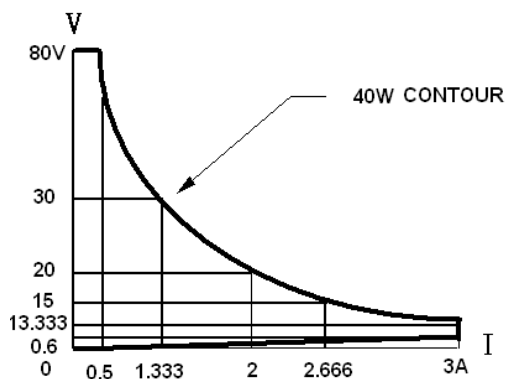
圖 1-4 3336F 0-80V/0-3A 40W 電子負載功率曲線圖
