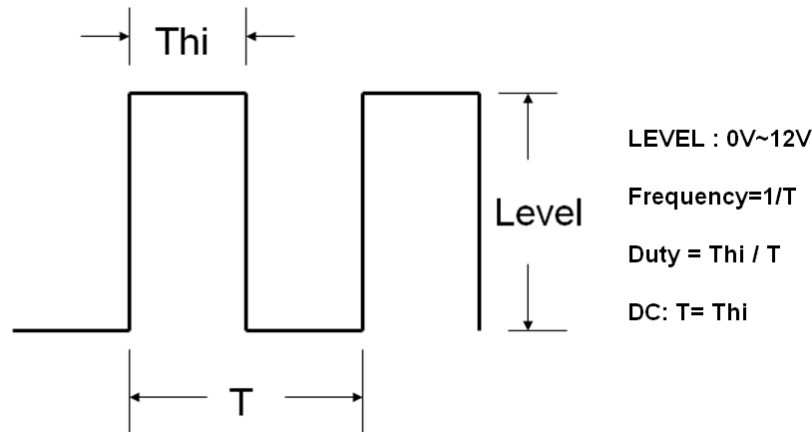
圖 3-3 3342G 系列電子負載 DIM 功能說明
