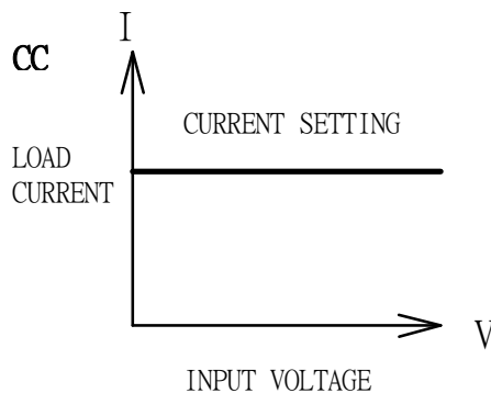
圖 1-3 固定電流模式特性圖
