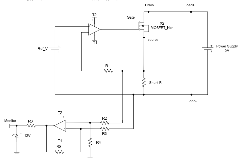
圖 3-4 3342G 系列 I-monitor 等效電路圖
