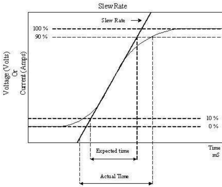
圖 1-9 回轉率(Slew Rate)曲線圖
