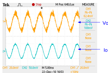
圖 4-9 LED Driver 的漣波
