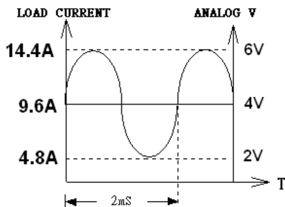
圖 3-7 負載電流之類比設定輸入
