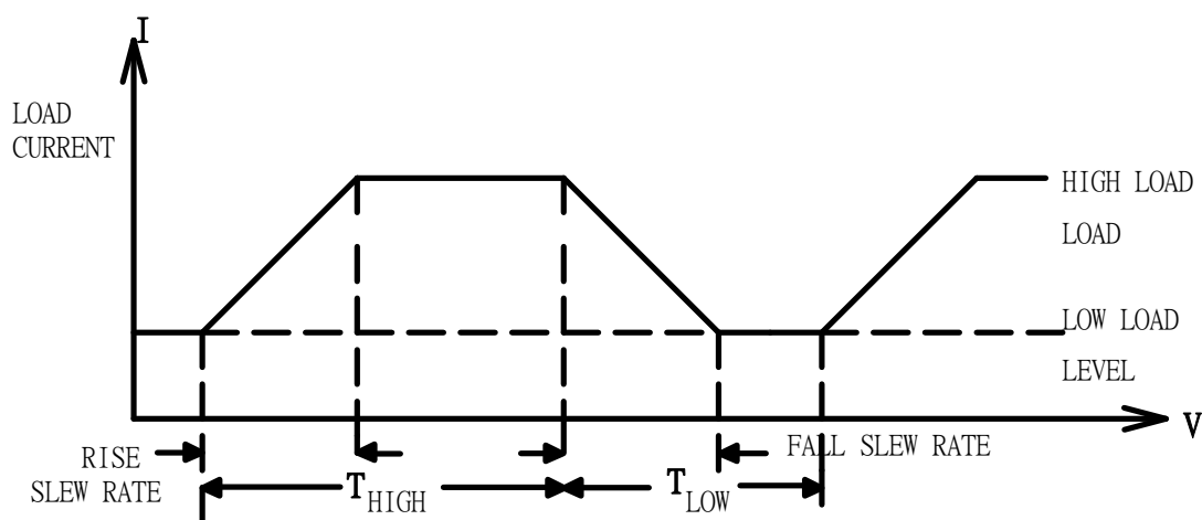
圖 1-8 動態負載模式特性圖
