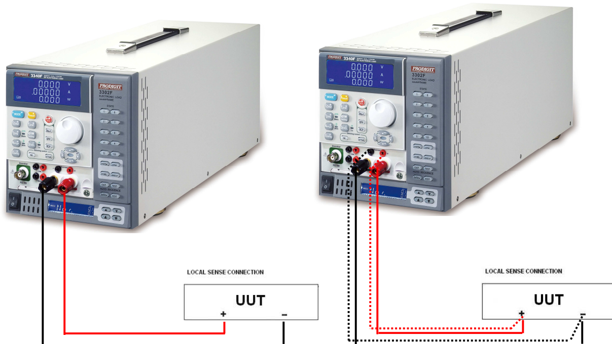
圖 3-2 典型的 3342G 系列電子負載連接方式
