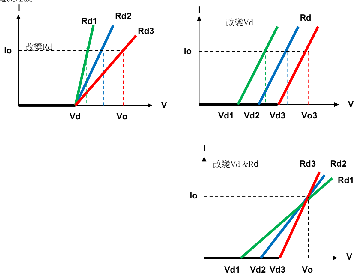
圖 4-12 LED MODE 操作模式之應用
