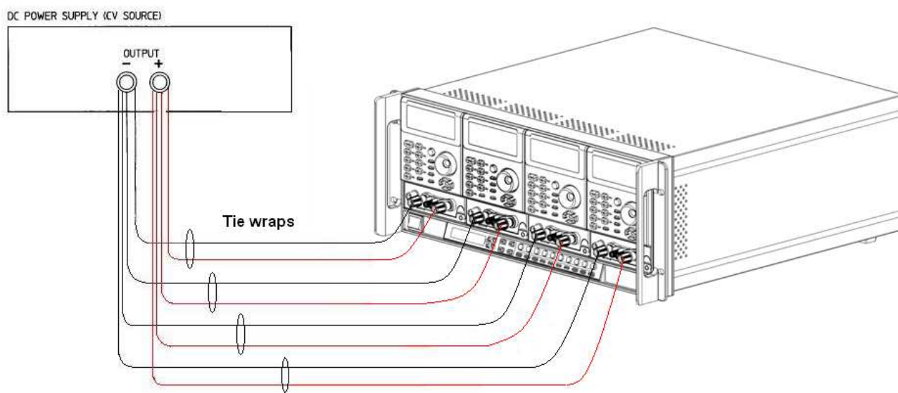
圖 4-14 電子負載多組並聯之連接圖
