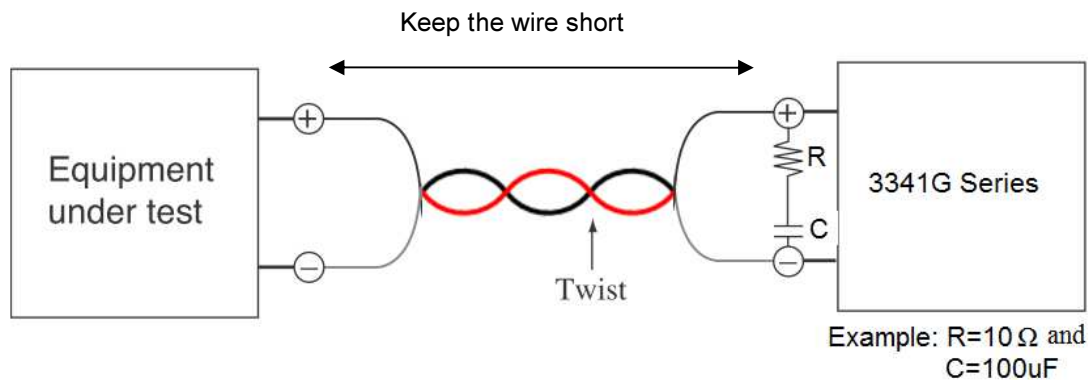
圖 2-5 接線長度
