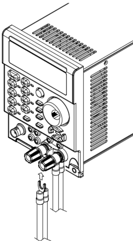
圖 3-8 Y型端子連接圖
