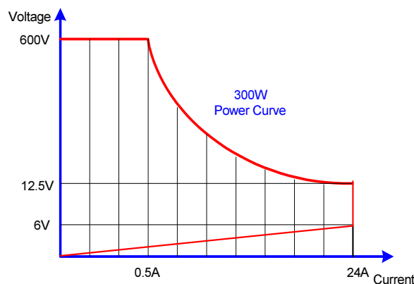
圖 1-2 3343G 0-600V/0-24A 300W 電子負載功率曲線圖
