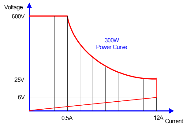
圖 1-1 3342G 0-600V/0-12A 300W 電子負載功率曲線圖
