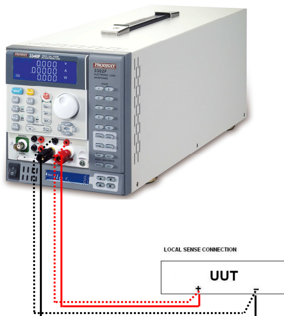
圖 4-2 遠地電壓檢知連接圖
