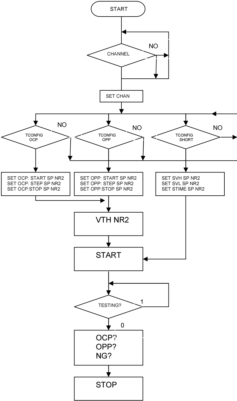
圖 4-16 3342G 系列電子負載 OCP、OPP、SHORT 操作流程圖
