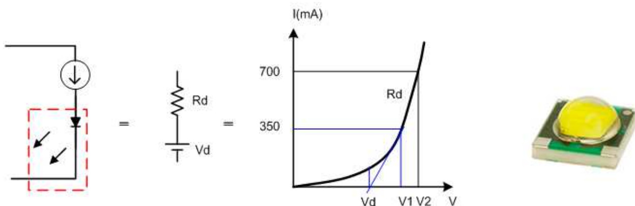
圖 4-8 LED 等效電路及特性曲線圖
