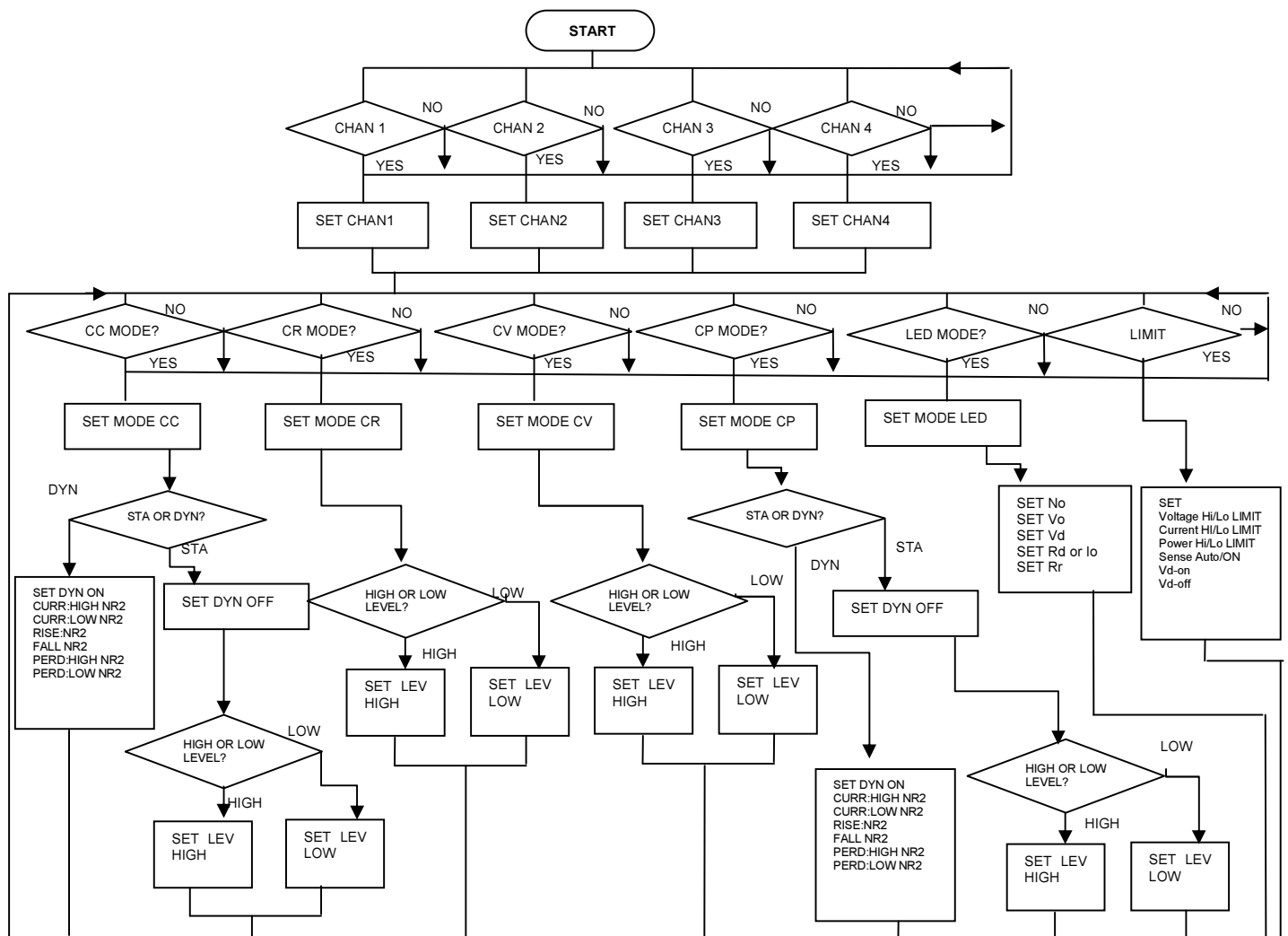
圖 2-3 3342G 系列電子負載操作流程圖
