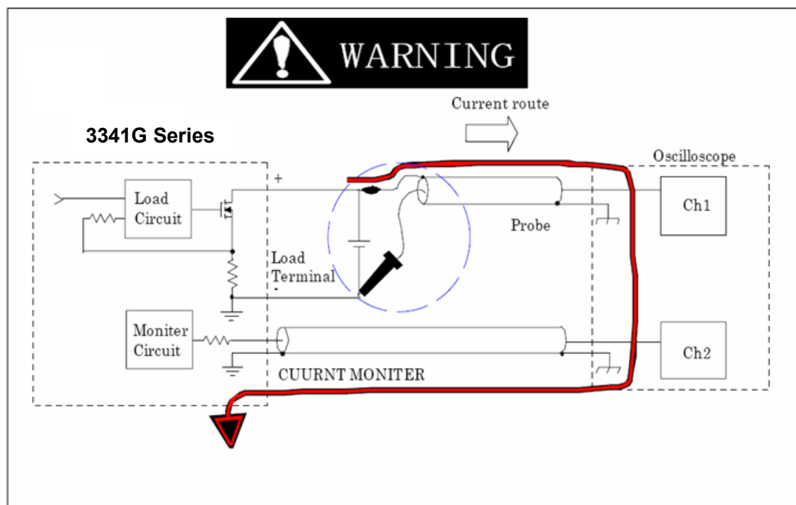
圖 3-5 示波器正確的連接圖
