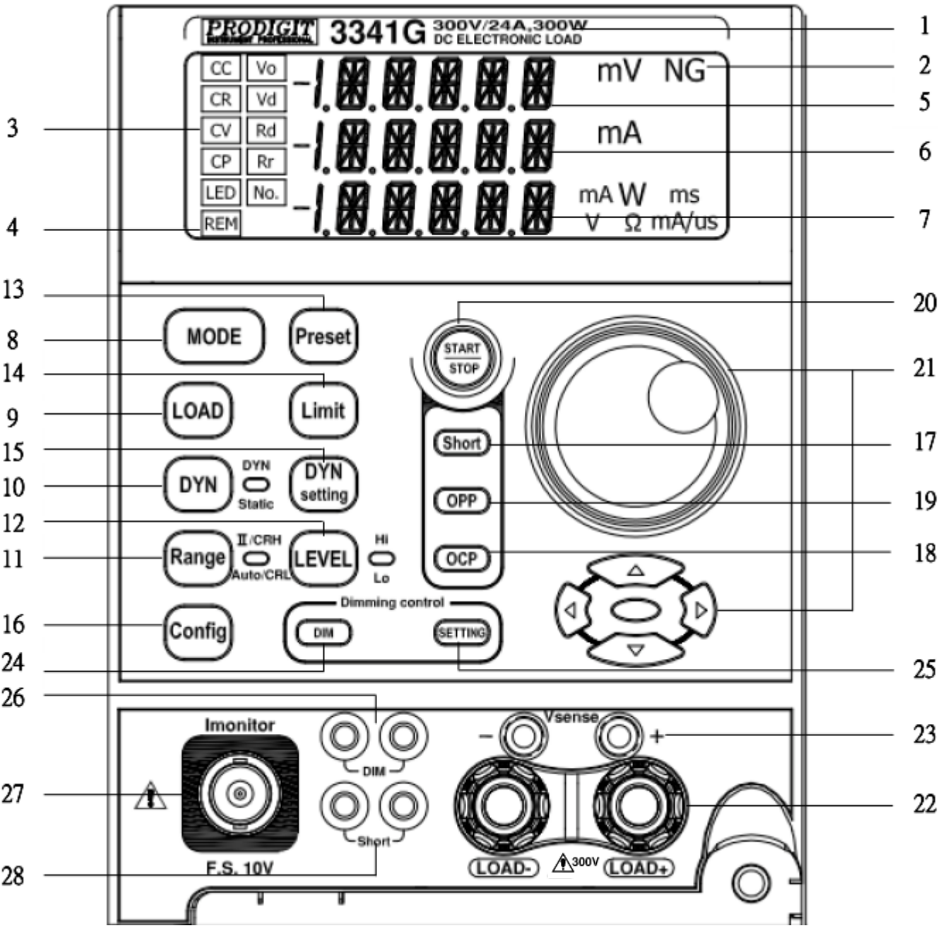
圖 3-1 前面板圖
