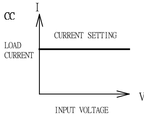
圖 1-4 固定電流模式特性圖
