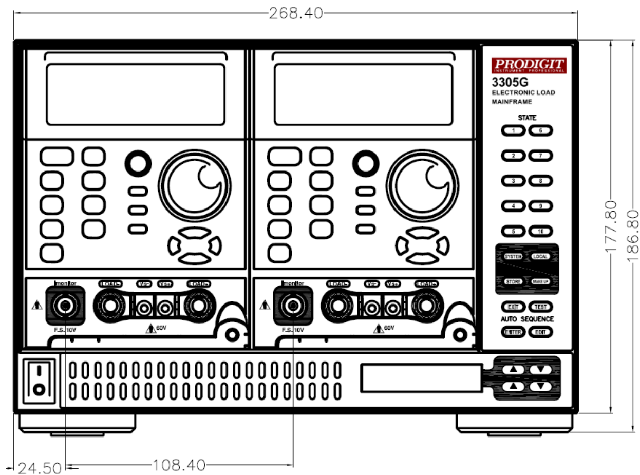
圖 3-1 3305G 前面板圖
