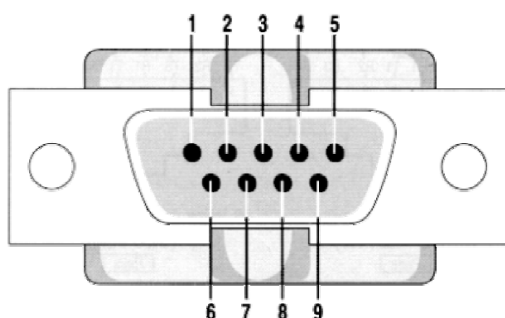
圖 4-1 後面板 RS232 介面連接圖
