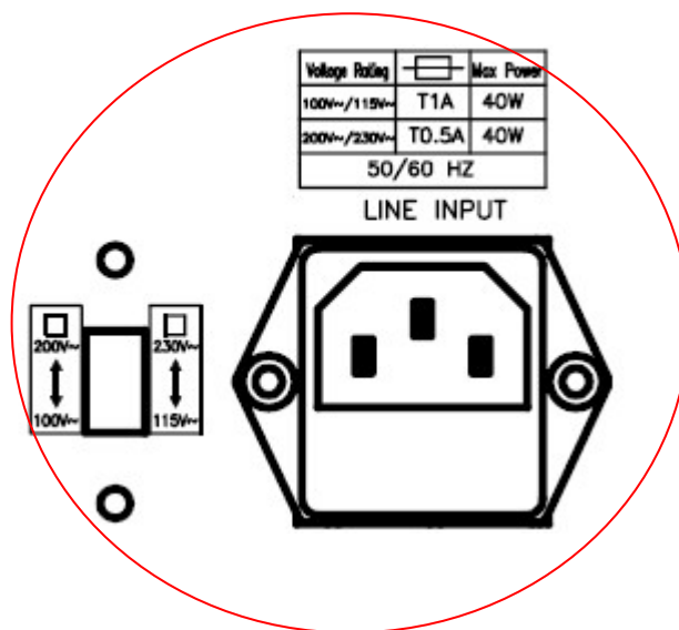
圖 2-1 電源設定圖
