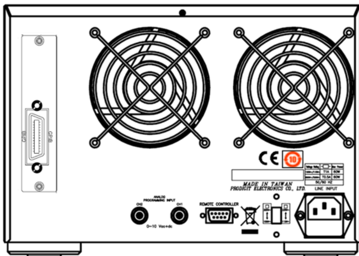
圖 3-3 3305G 後面版圖
