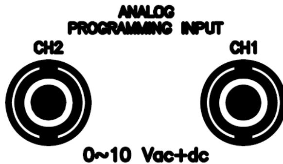
圖 2-10 3305G 類比信號設定輸入介面
