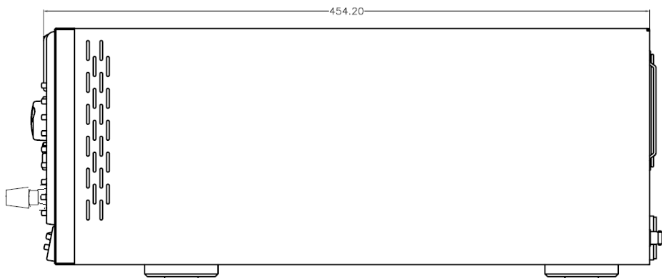
圖 3-2 3305G 側面圖
