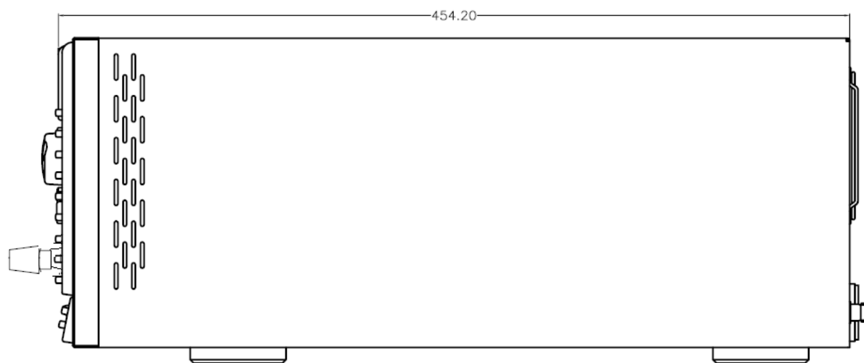
圖 3-2 3302G 側面圖
