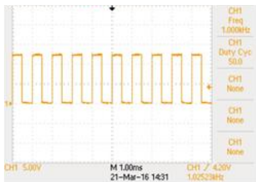
數位式PWM調光信號
