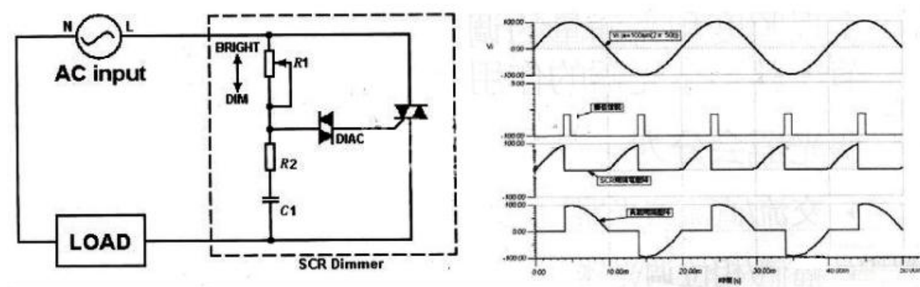
圖一 傳統的類比式調光器
