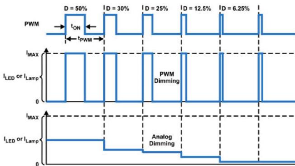
圖三 採用類比調光及 PWM 調光時的燈光或 LED 電流
