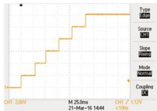
類比式 2V到12V 調光信號
