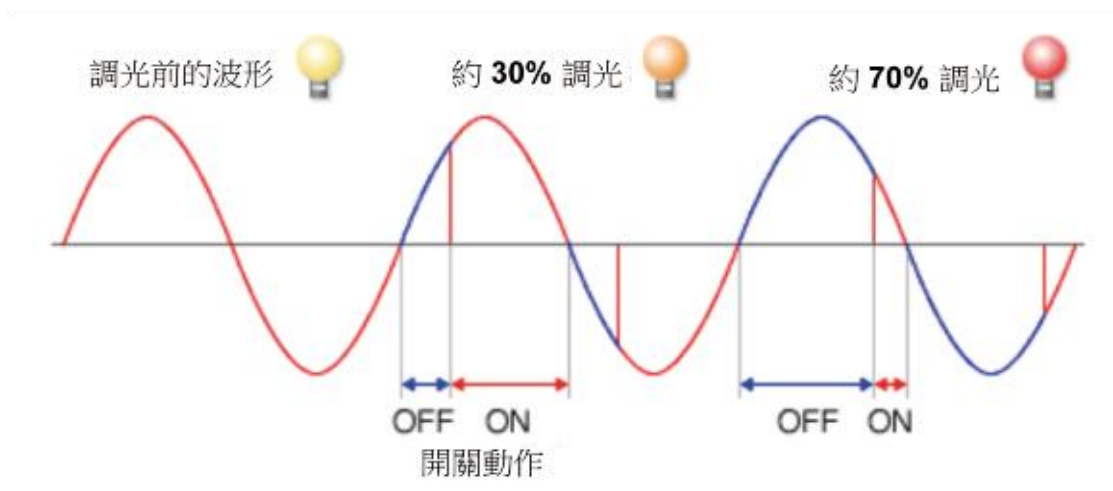
圖一 傳統的類比式調光器
