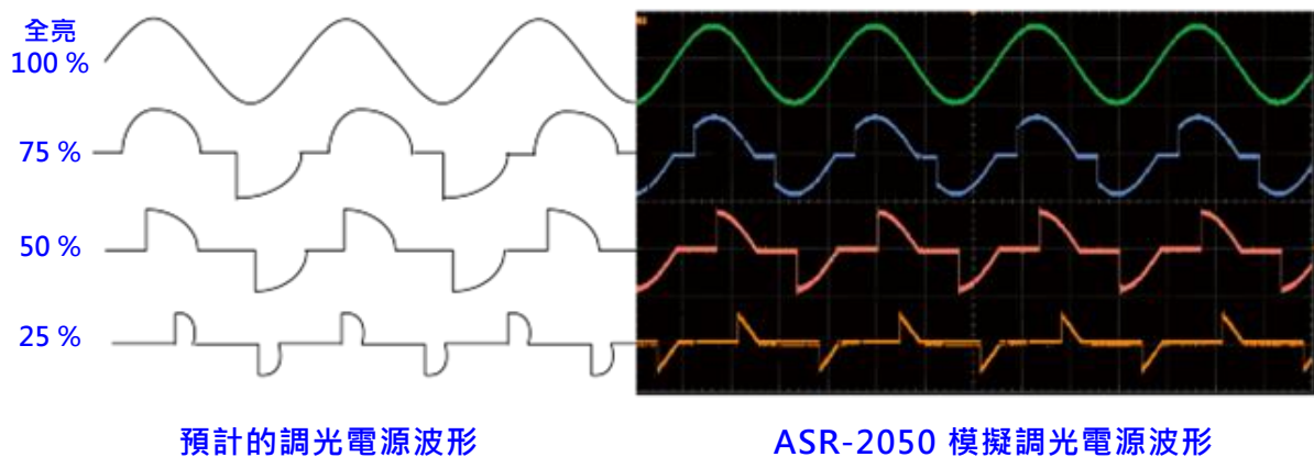
圖四 ASR 系列交直流電源模擬傳統調光器 ( TRIAC )
