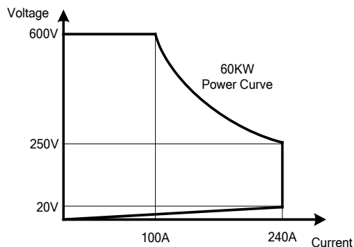
1-1.2 36260A高功率電子負載功率曲線圖
