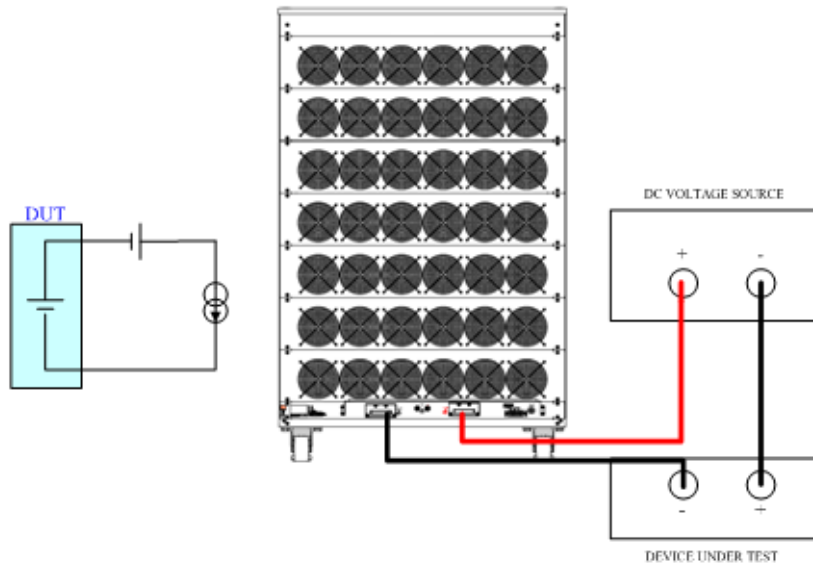
圖 5-11 高功率電子負載最低工作電壓為 0V 時的連接圖
