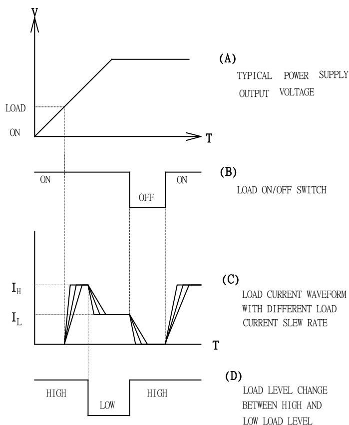
圖 2-8 負載電流波形與 LOAD ON/OFF 開關
