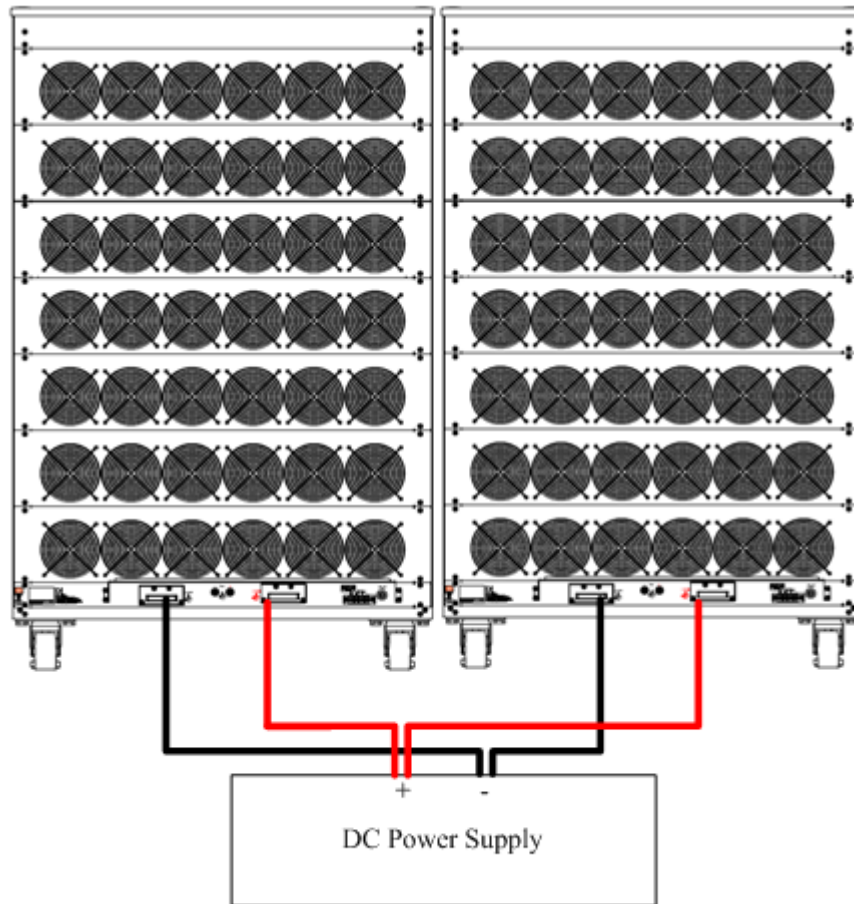
圖 5-12 電子負載多組並聯之連接圖
