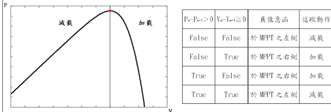
圖 5-14 擾動觀察法動作方式
