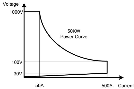
圖 1-1.3 36350A 高功率電子負載功率曲線圖
