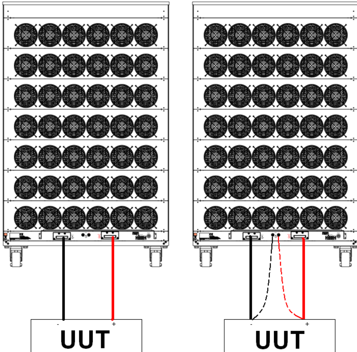
圖 3-4 典型 36000A 系列高功率電子負載連接方式
