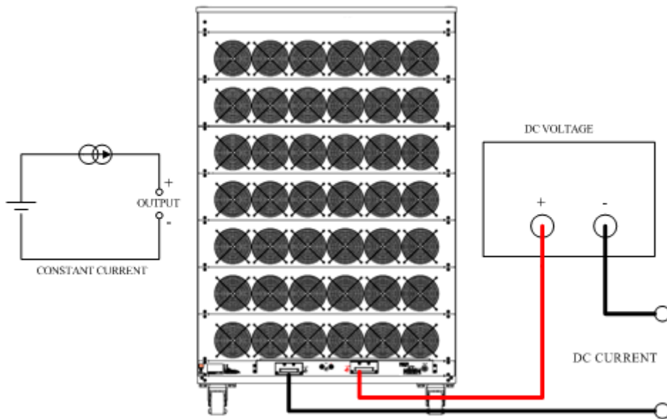
圖 5-10 固定電流源之連接圖
