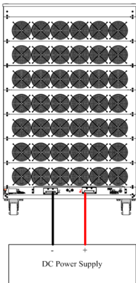
圖 5-1 本地電壓檢知連接圖
