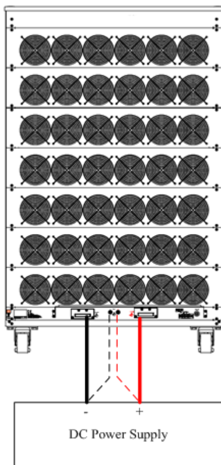
圖 5-2 遠地電壓檢知連接圖
