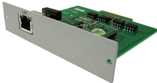
圖 2-6 36000A 系列 LAN 連接埠圖
