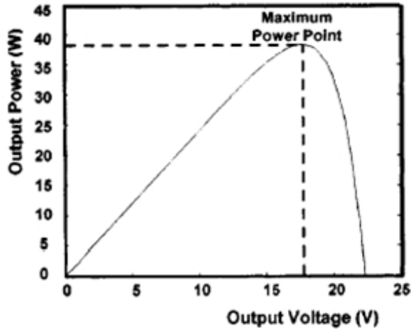
圖 5-13 最大功率點追蹤
