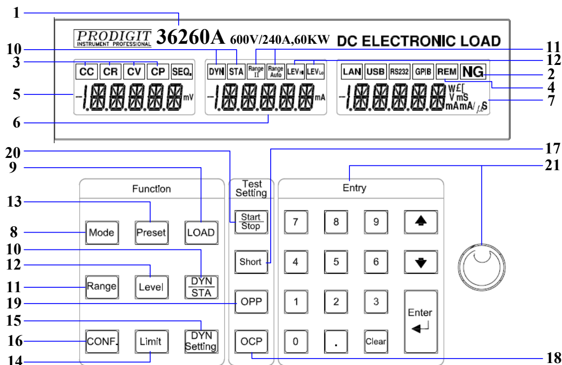
圖 3-3 36000A 系列高功率電子負載之面板圖
