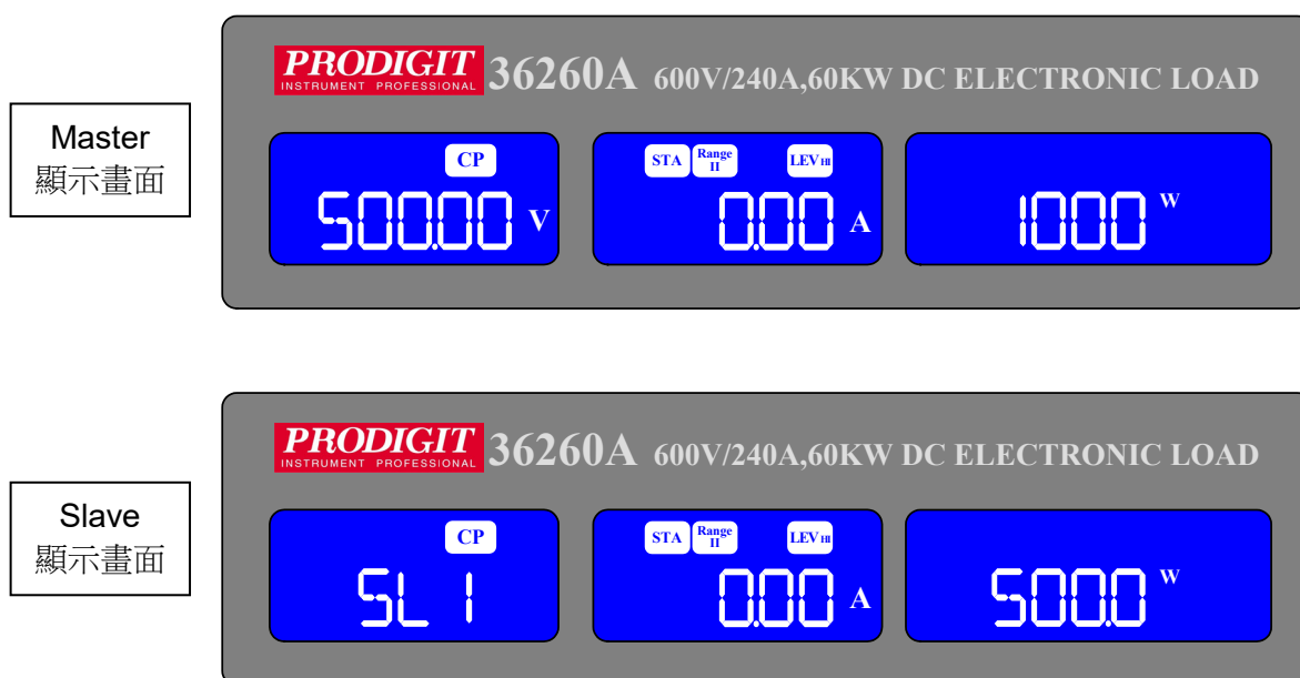
圖 CP Set 1000W
