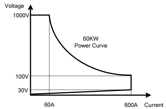
1-1.4 36360A 高功率電子負載功率曲線圖
