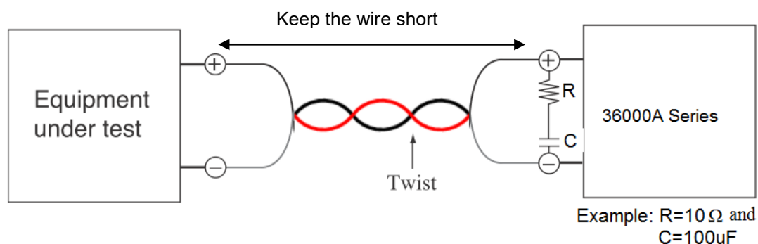
圖 2-10 接線長度
