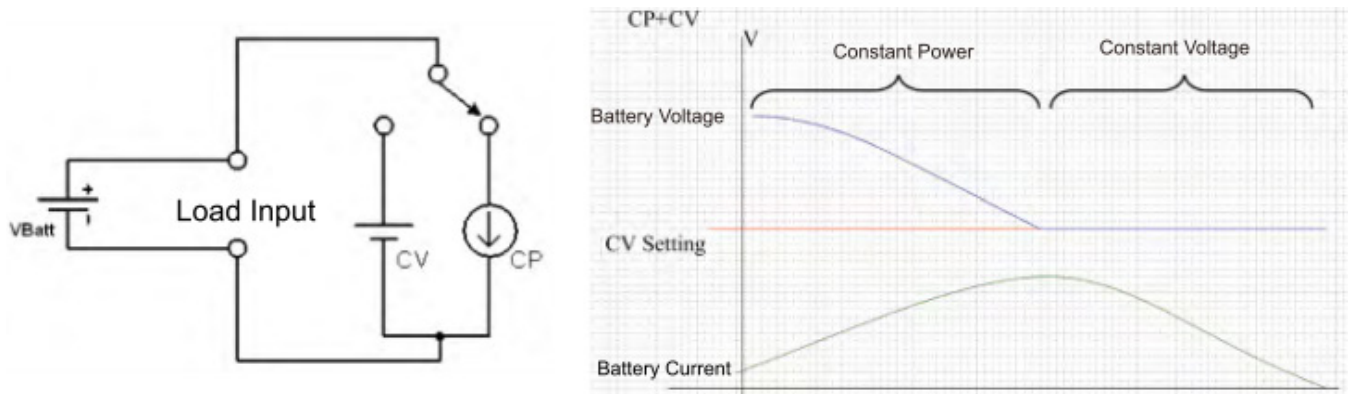
圖 5-9 CP 轉換為 CV 操作模式之應用
