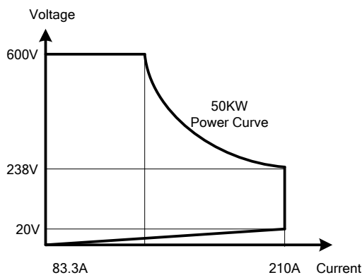
圖 1-1.1 36250A高功率電子負載功率曲線圖
