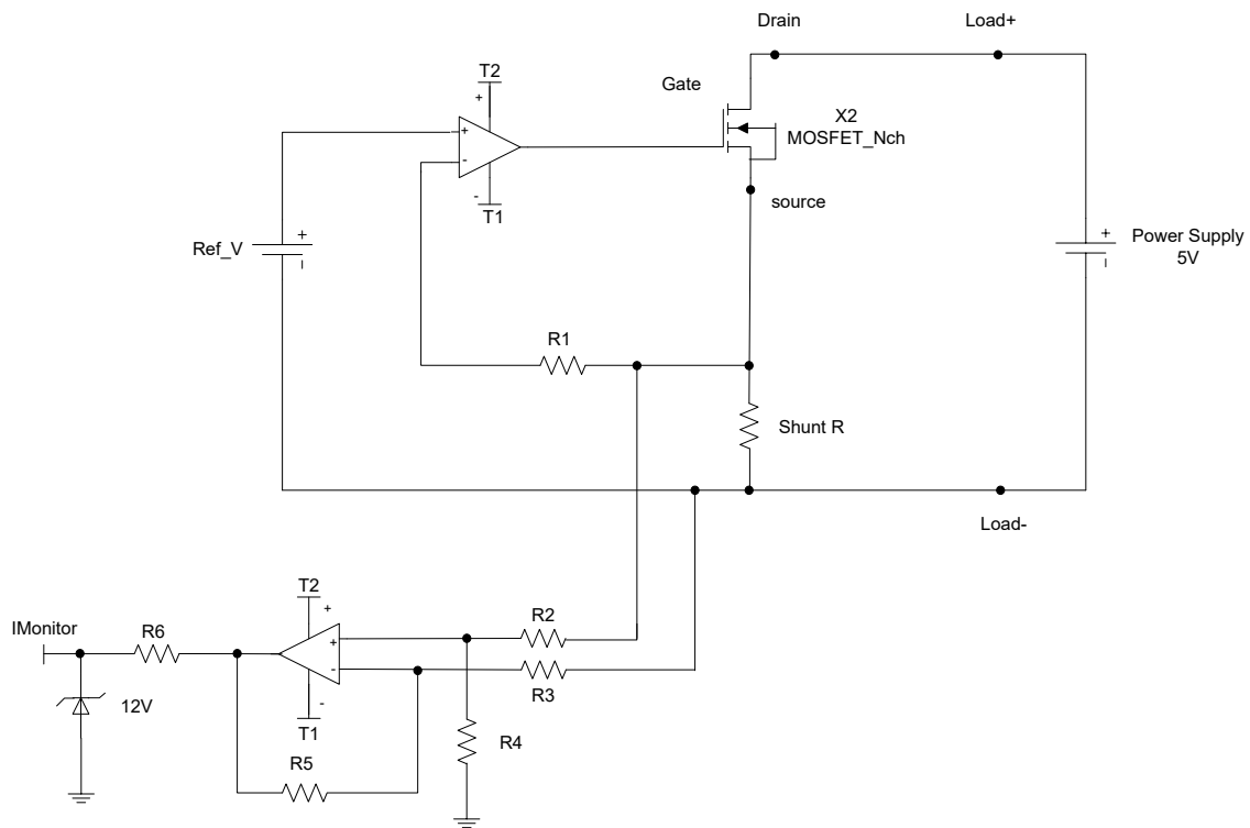
圖 3-5 36000A 系列 I-monitor 等效電路圖
