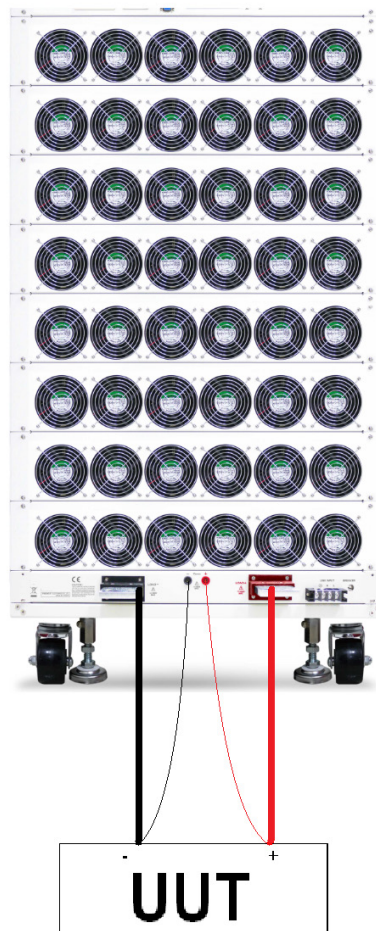
圖 5-2 遠地電壓檢知連接圖
