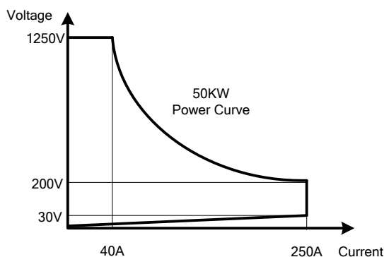
圖 1-1.1 36350E高功率電子負載功率曲線圖
