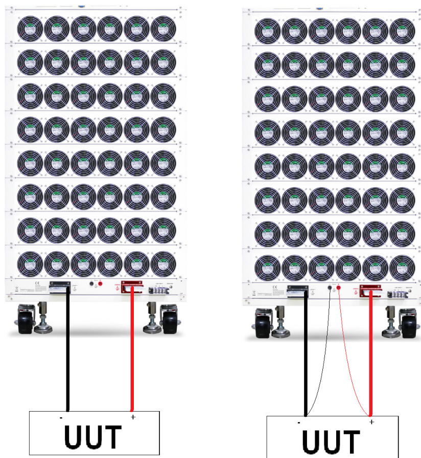
圖 3-4 典型 36000E 系列高功率電子負載連接方式
