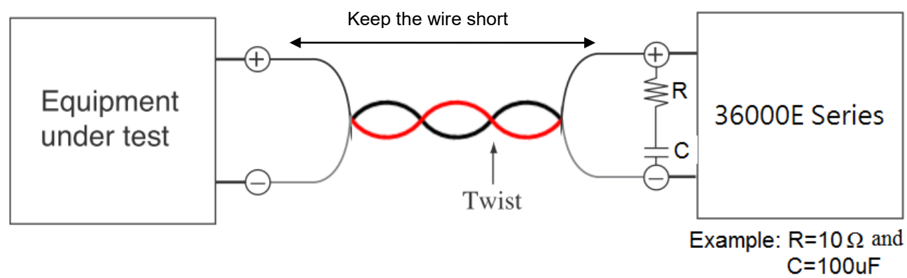
圖 2-10 接線長度
