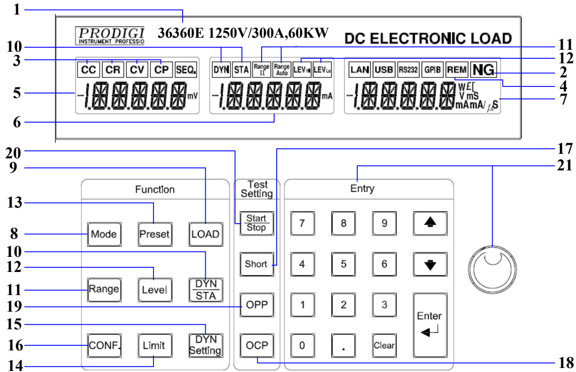
圖 3-3 36000E 系列高功率電子負載之面板圖
