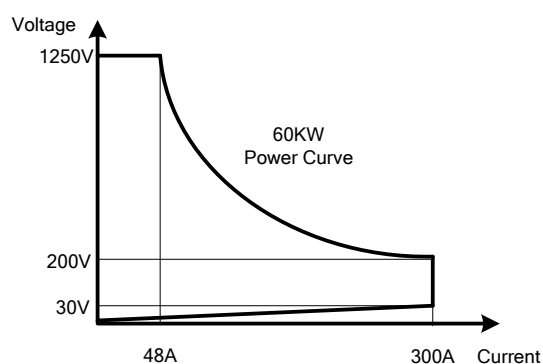
1-1.2 36360E高功率電子負載功率曲線圖
