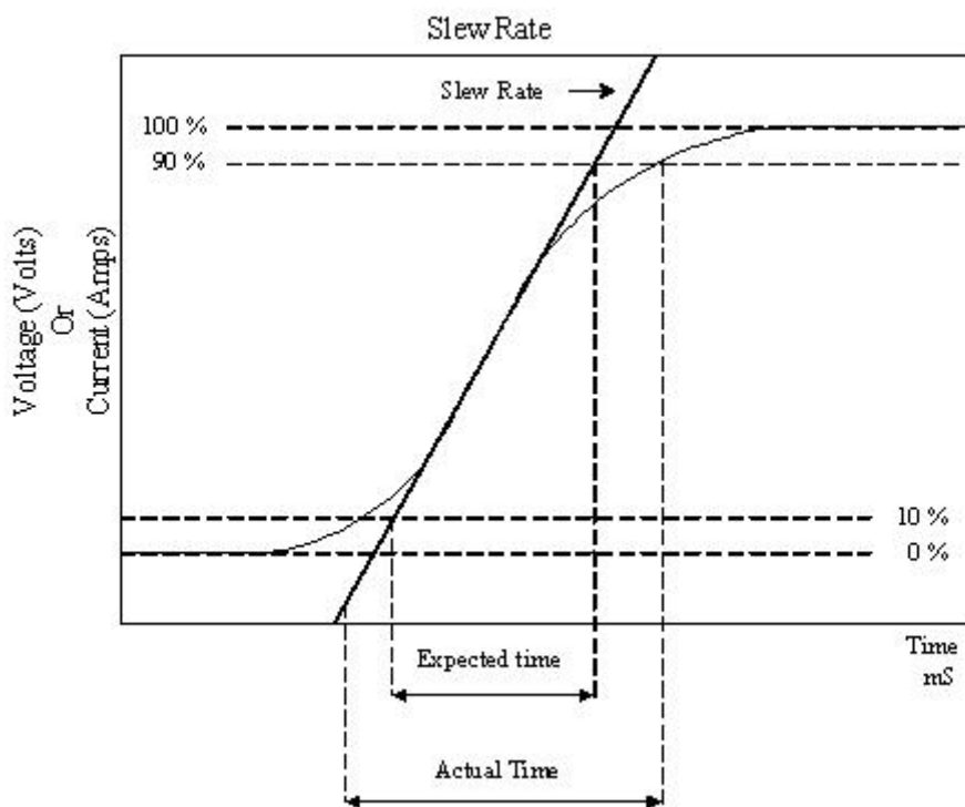
圖 1-7 回轉率 (Slew Rate) 圖
