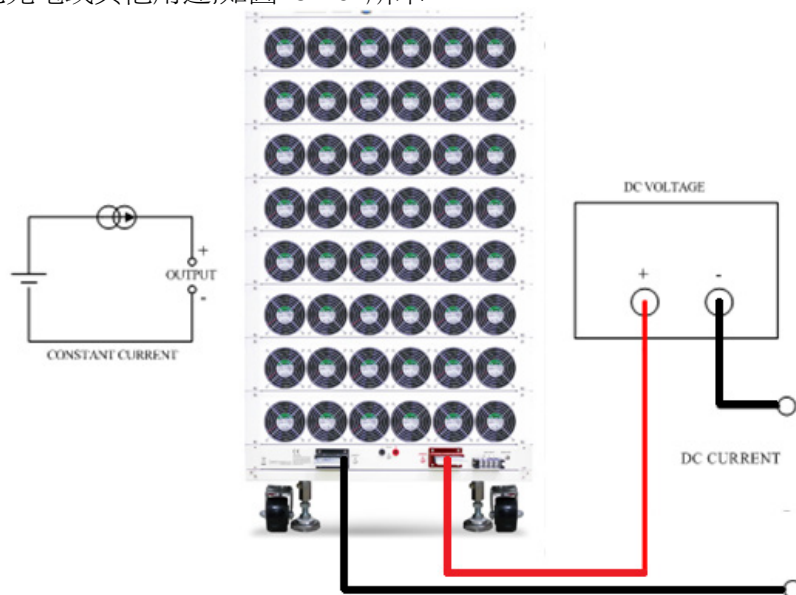
圖 5-10 固定電流源之連接圖
