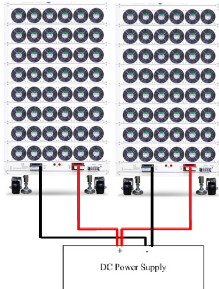
圖 5-12 電子負載多組並聯之連接圖
