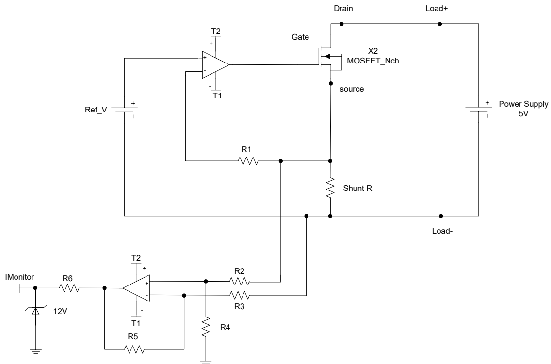
圖 3-5 36000E 系列 I-monitor 等效電路圖
