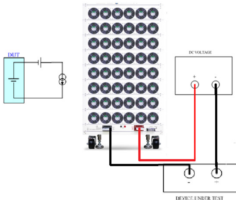
圖 5-11 高功率電子負載最低工作電壓為 0V 時的連接圖
