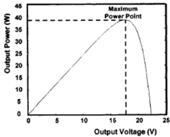
圖 5-13 最大功率點追蹤
