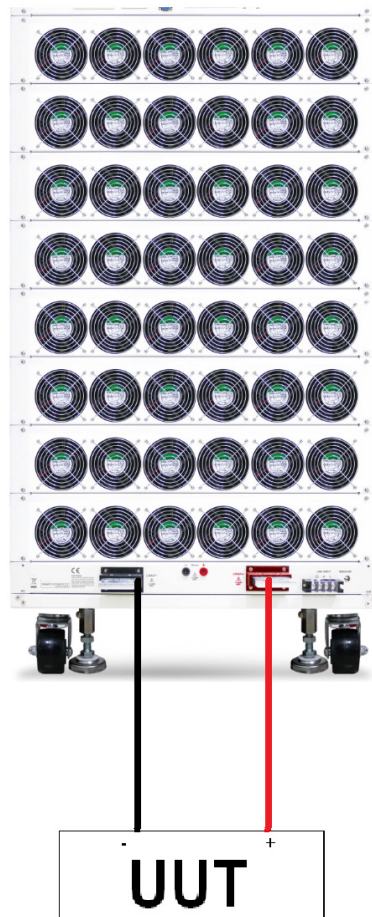
圖 5-1 本地電壓檢知連接圖
