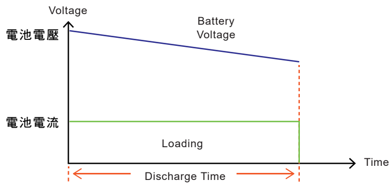
圖 8：設定放電時間電池放電測試
