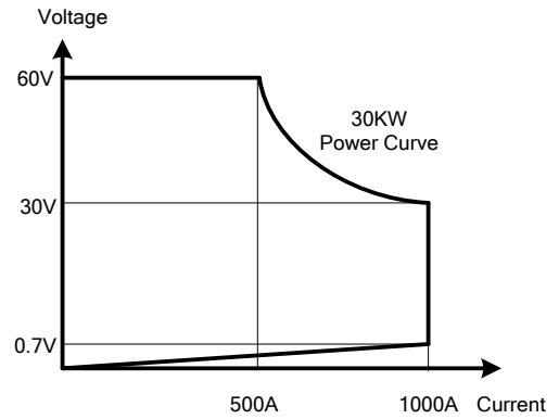
圖 1-1.6 34130A高功率電子負載功率曲線圖
