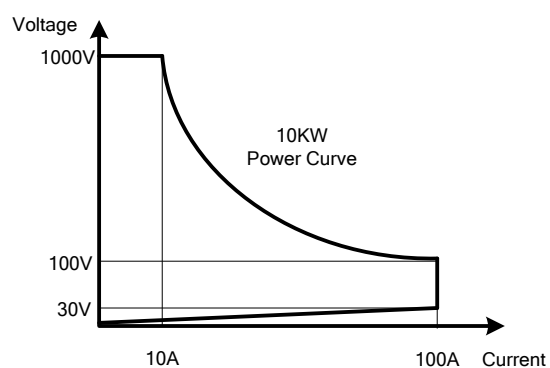
1-1.18 34310A高功率電子負載功率曲線圖
