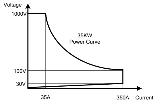
圖 1-1.23 34335A高功率電子負載功率曲線圖
