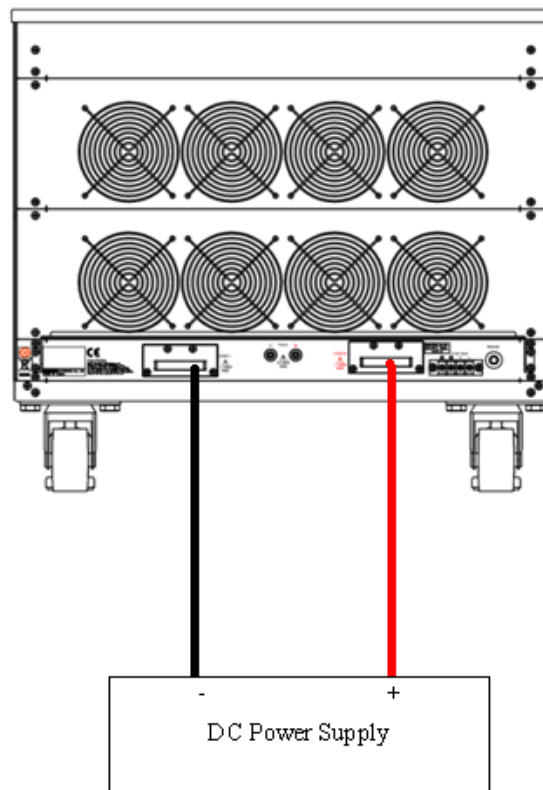
圖 5-1 本地電壓檢知連接圖
