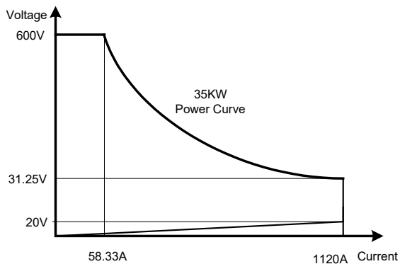
圖 1-1.15 34235A高功率電子負載功率曲線圖
