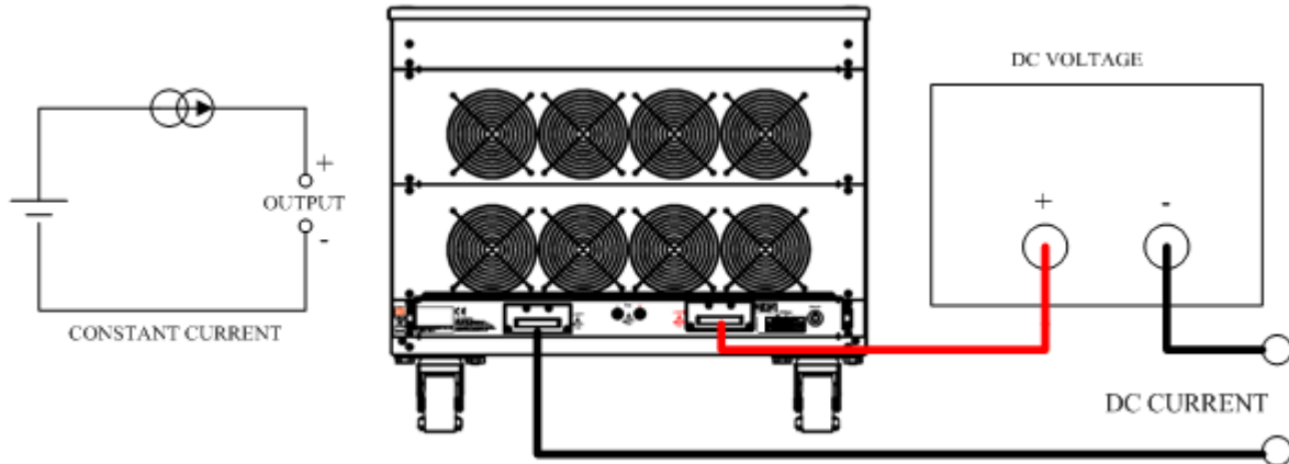
圖 5-10 固定電流源之連接圖
