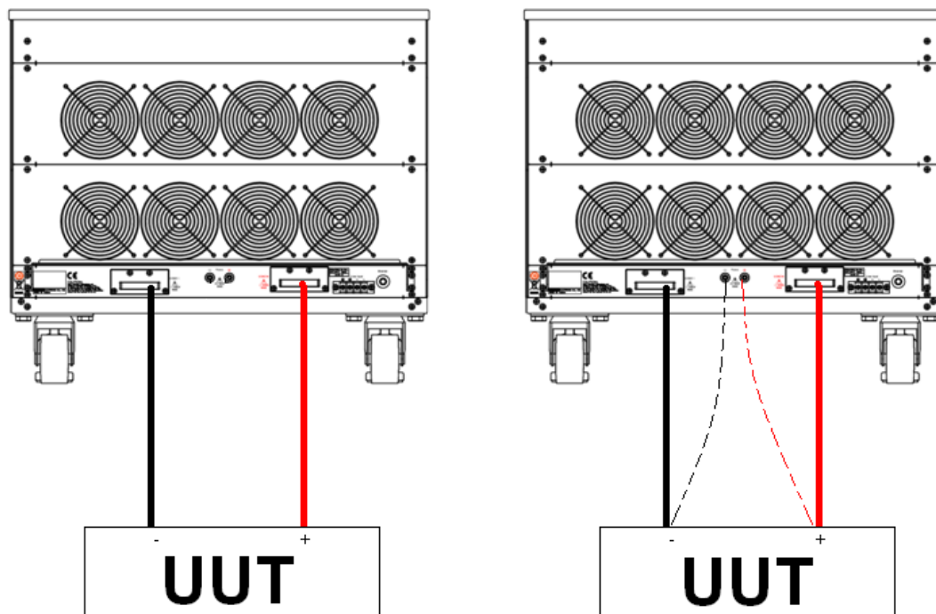
圖 3-4 典型 34000A 系列高功率電子負載連接方式
