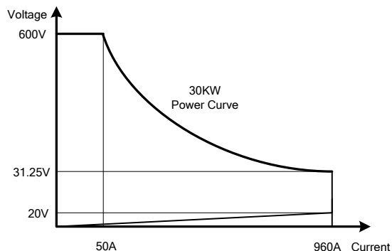
1-1.14 34230A高功率電子負載功率曲線圖
