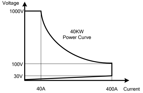
圖 1-1.24 34340A高功率電子負載功率曲線圖
