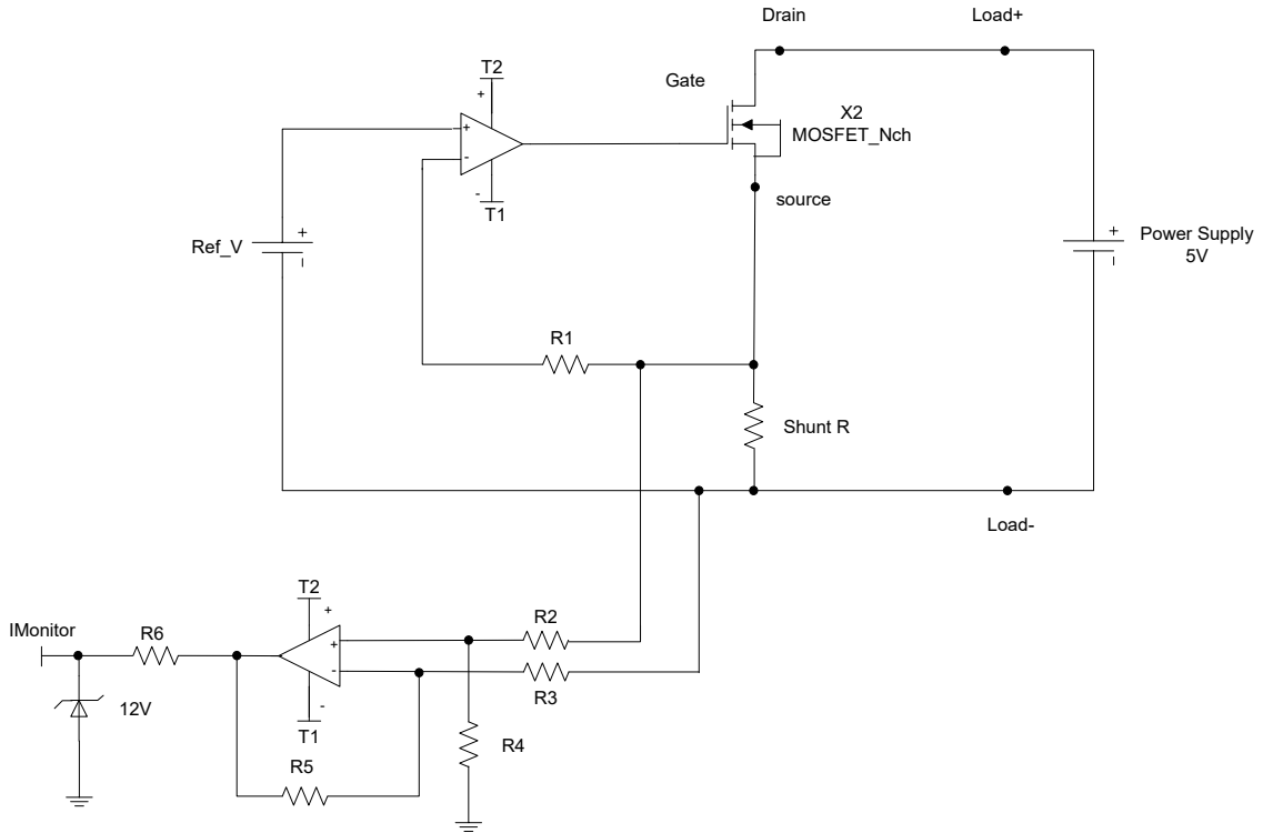
圖 3-5 34000A 系列 I-monitor 等效電路圖
