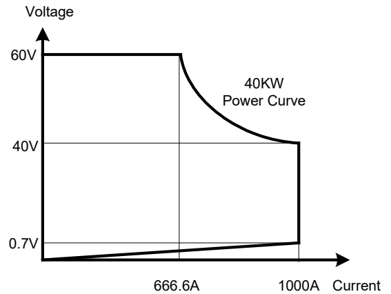
圖 1-1.8 34140A高功率電子負載功率曲線圖
