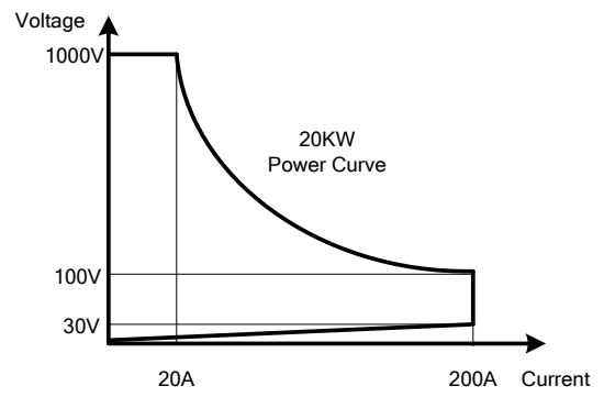
圖 1-1.20 34320A高功率電子負載功率曲線圖
