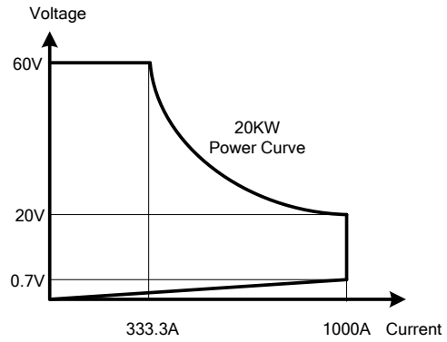
圖 1-1.4 34120A高功率電子負載功率曲線圖
