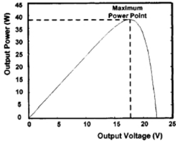
圖 5-11 最大功率點追蹤
