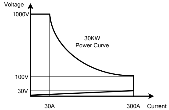
圖 1-1.22 34330A高功率電子負載功率曲線圖
