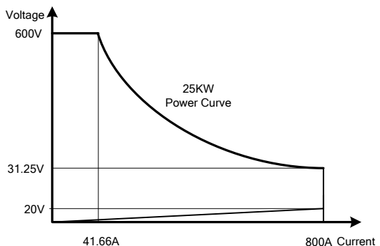
圖 1-1.13 34225A高功率電子負載功率曲線圖
