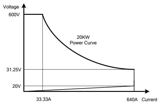
1-1.12 34220A高功率電子負載功率曲線圖
