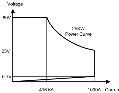
圖 1-1.5 34125A高功率電子負載功率曲線圖
