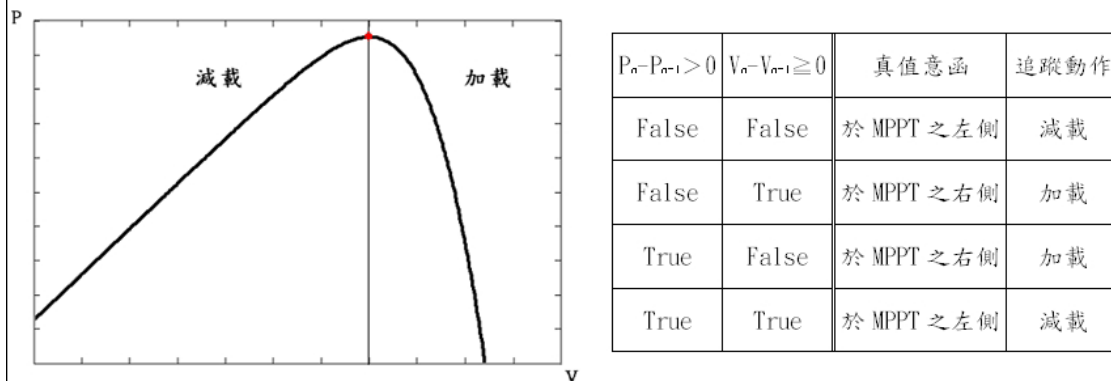
圖 5-12 擾動觀察法動作方式
