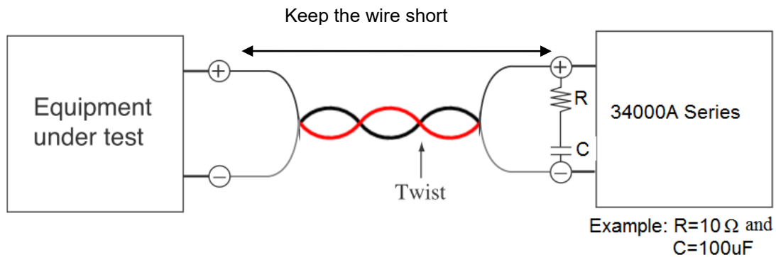
圖 2-10 接線長度
