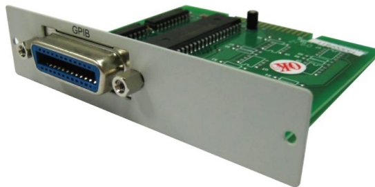
圖 2-4 34000A 系列高功率電子負載 GPIB 介面
