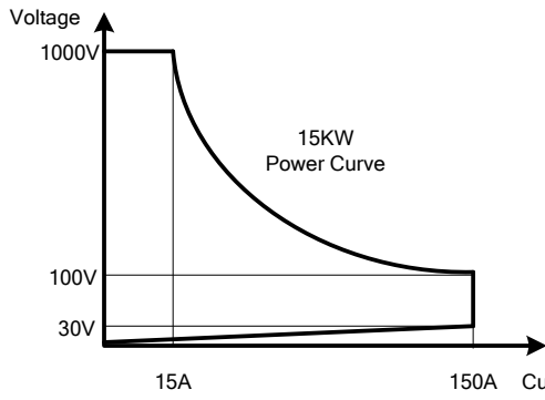
圖 1-1.19 34315A高功率電子負載功率曲線圖
