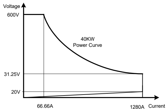
1-1.16 34240A高功率電子負載功率曲線圖
