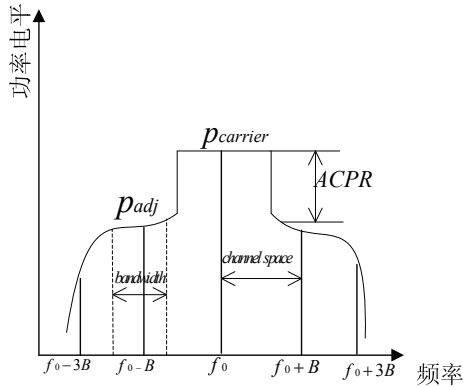
图 7-2 ACPR 的定义
