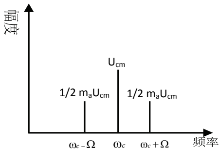
图 5-3 调幅波的频谱
