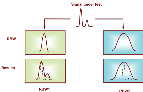
图 5 不同的 RBW 的 影响 (2)
