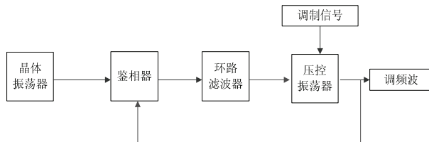
图 6-2 GRF-1300 调频 原理
