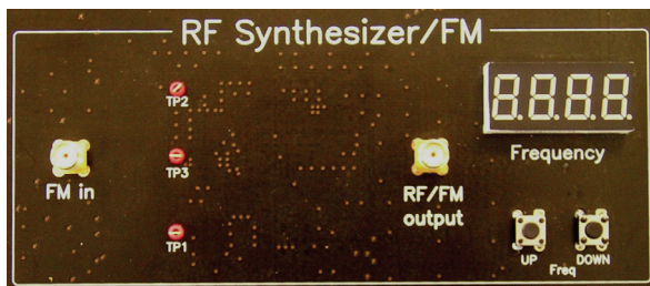
图 A-5 RF Synthesizer/ FM 模块
