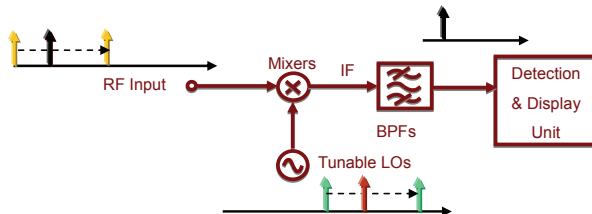
图 3 RBW 过滤器
