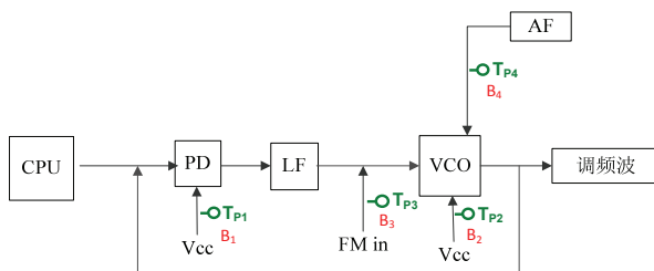
图 A-7 各测试点对应的 电路位置
