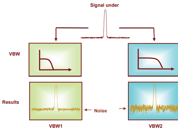
图 8 对不同的 VBW 的影响
