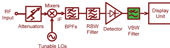
图 7 在系统里的 VBW 滤波器
