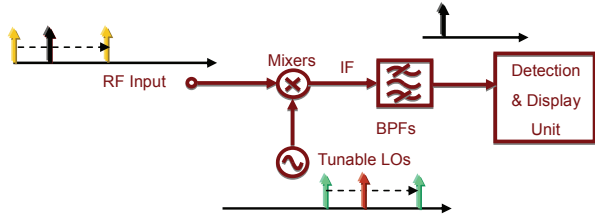
图 1 宽带接收者的基本结构
