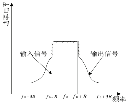
图 7-1 射频频率放大器 输入输出
